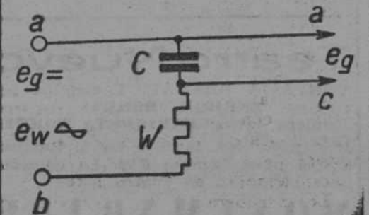
Fig. 5.—Fuente de corriente supuesta
