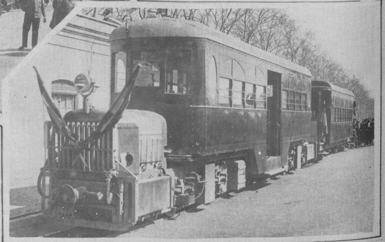
Molores de la casa Krupp y coches construidos en la casa Enrique Quintana. Automotor con su remolque.
