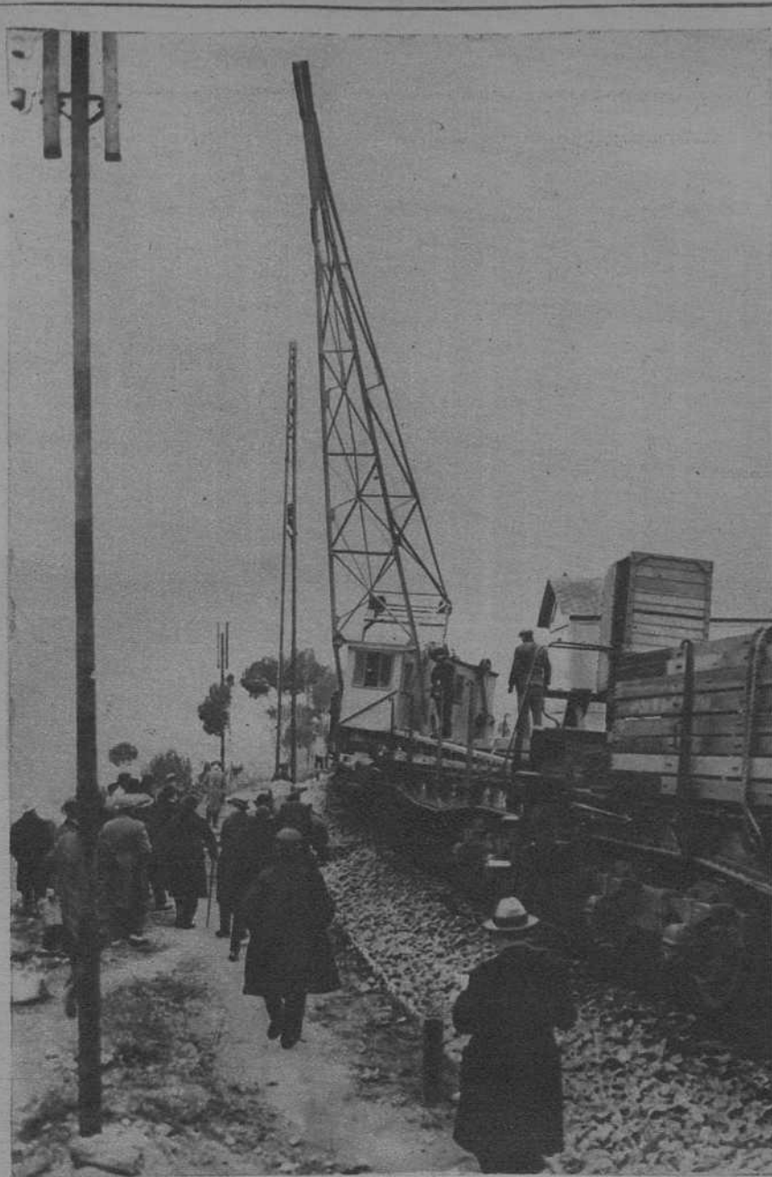
Obras de electrificación de la línea Barcelona-Manresa: tren para la colocación de postes.
