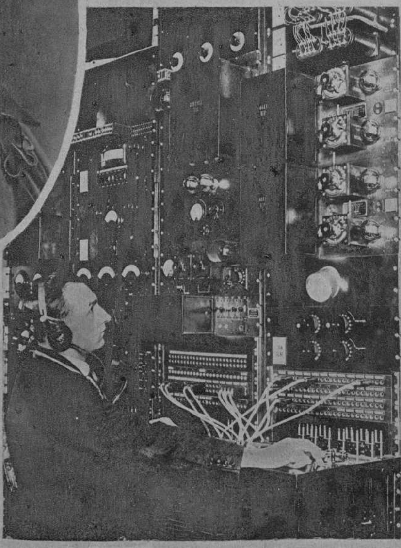
LONDRES Y NUEVA YORK EN COMUNICACION POR RADIO Instalación que se ha utilizado para la comunicación por radiotelefonía entre Londres y Nueva York; costará 15 libras (475 pesetas) la conferencia de tres minutos (Fot. Vidal)
