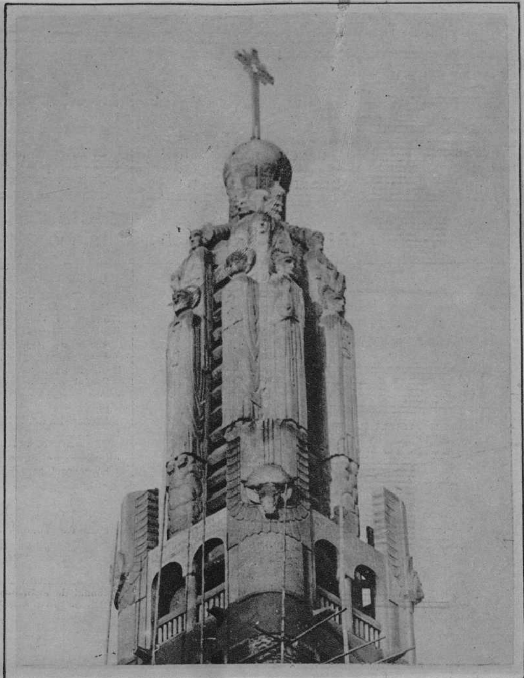
FRANCIA.—UNA OBRA GIGANTESCA: DOS VISTAS DE LA NUEVA IGLESIA QUE SE ESTA CONSTRUYENDO EN VILLEMONTBLE, BAJO LA DIRECCION DEL ARQUITECTO TOURNON. EL CAMPANARIO, CONSTRUIDO ENTERAMENTE DE CEMENTO ARMADO, MIDE UNA ALTURA DE 54 METROS POR 18 DE ANCHURA, Y ESTA CORONADO DE COLOSALES ESTATUAS (Fot. Consorcio)
