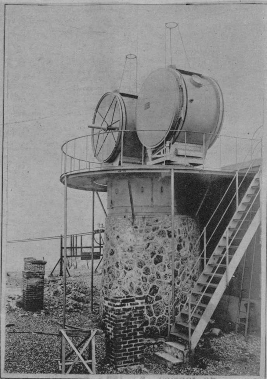
PARIS.—En el Mont-Valérien acaba de inaugurarse este faro, que se considera como el de mayor potencia del mundo (Fot. Consorcio)
