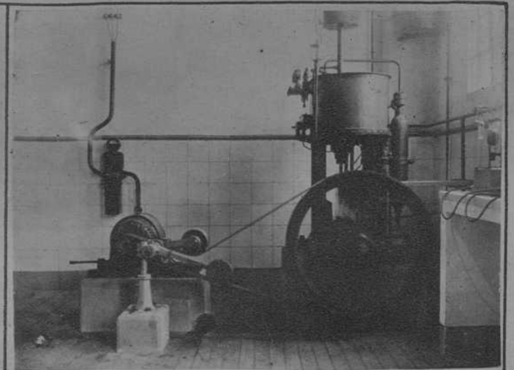
Compresor de oxígeno
