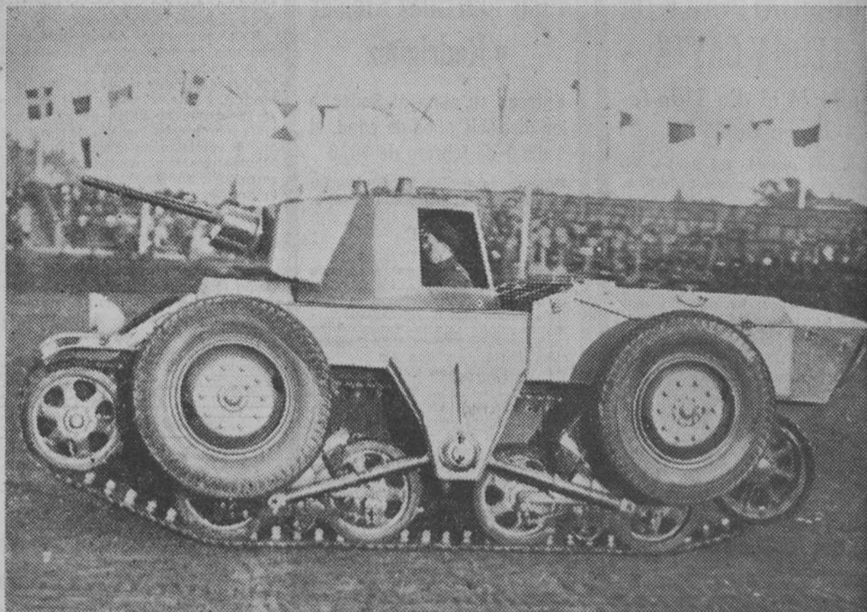
Un nuevo tanque sueco. En dieciocho segundos cambia el sistema de marcha. Sobre las ruedas alcanza una velocidad de 75 kilómetros, y de 40 como «auto-oruga» (Foto Vidal)
