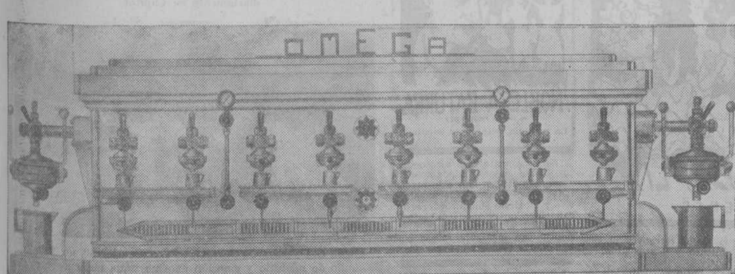
Fotografía de la máquina cafetera OMEGA RECTANGULAR, de ocho canillas individuales y dos canillas múltiples, fabricada en los
