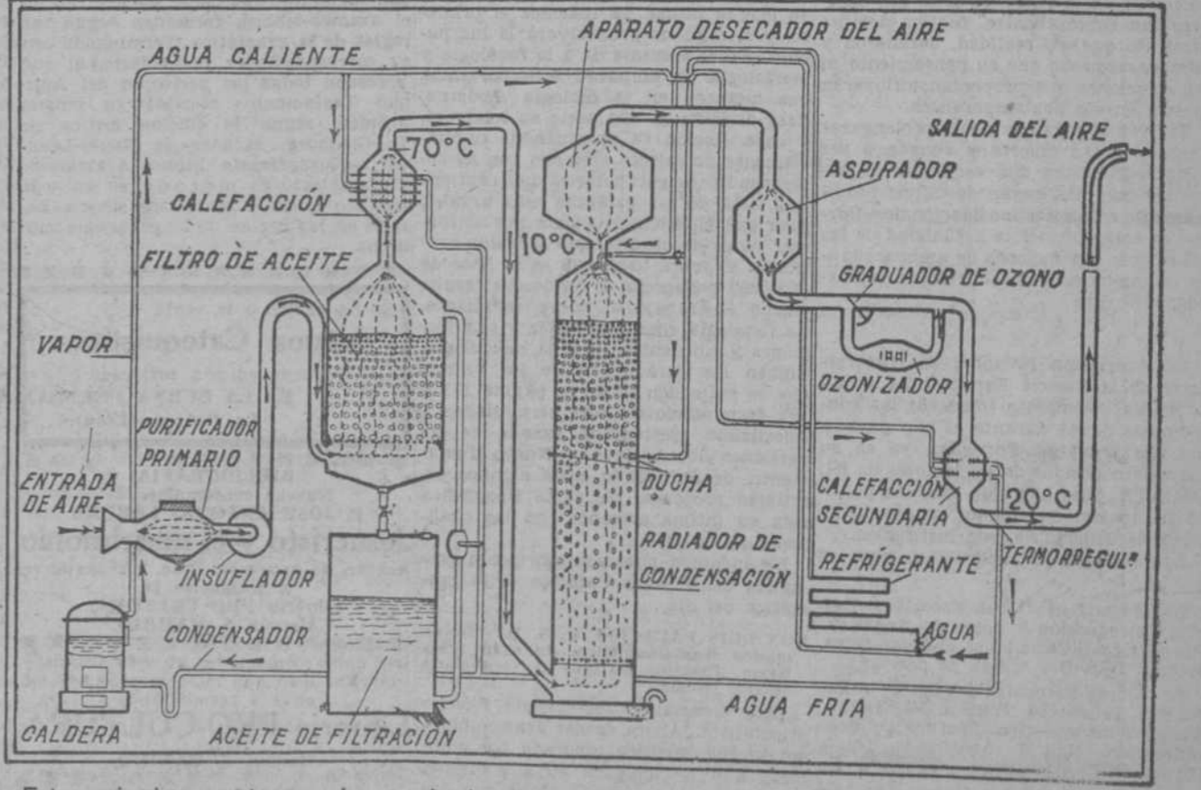
Esta serie de aparatos son los que ha inventado Móscicki para filtrar, purificar, humidificar, ozonizar y templar el aire de las habitaciones
