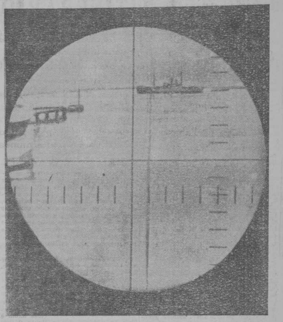
Fotografía obtenida a través del periscopio de un submarino. El campo visual del observador está dividido en cuatro partes, por dos diámetros, uno vertical y otro horizontal. Cada cuadrante se subdivide en determinadas graduaciones, las cuales permiten apreciar las distancias y la situación de los barcos que están en la superficie del mar.
