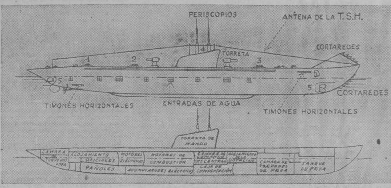
Diagrama de un submarino del tipo de los construídos en los últimos años de la guerra. 1, 2, 3 y 4, escotillas; 5, bocas de los tubos lanzatorpedos.
