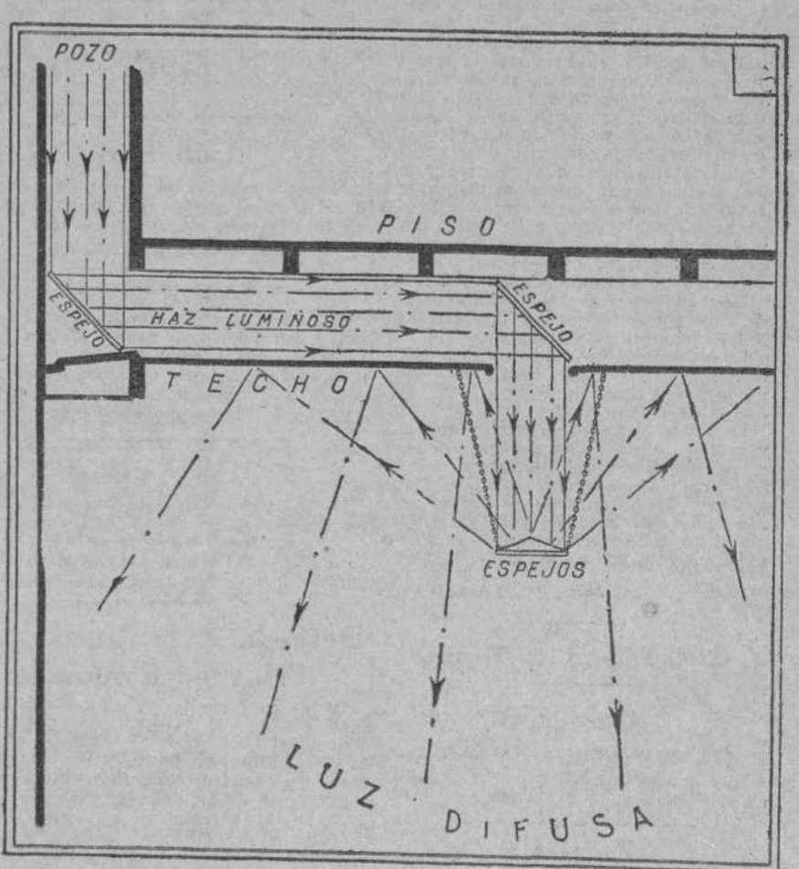
Fig. 5. La luz solar entra canalizada entre paredes y techos hasta una lámpara colgante formada de espejos
