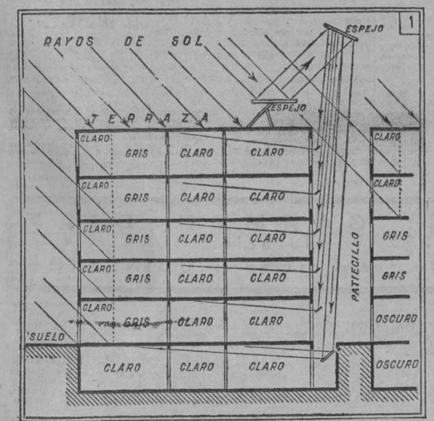
Fig. 1. Los rayos solares, reflejados en dos espejos, penetran hasta los sótanos más débregos
