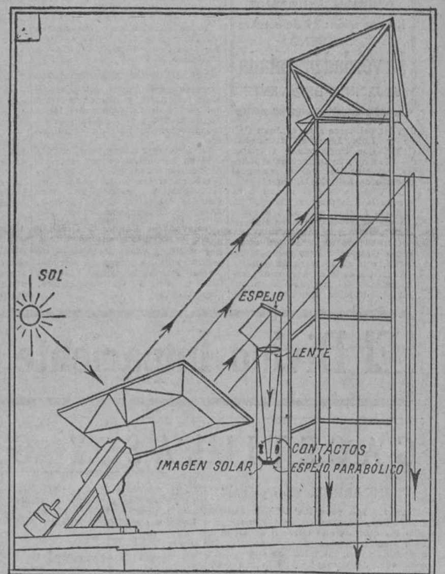
Fig. 3. El "tubo-director", que parece una cabeza de jirafa, lleva en su interior todo el secreto del mecanismo con el que el mismo sol gobierna los movimientos del espejo que primero refleja los rayos que él envía
