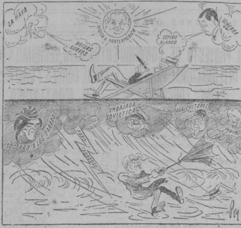
EL TIEMPO HACE UNOS MESES Y EL TIEMPO QUE HACE AHORA
