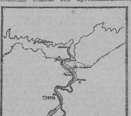
Copia hecha sobre el Mapa Militar Itinerario de España, formado por el Cuerpo de Estado Mayor del Ejército en 1920, en la parte correspondiente al croquis publicado en EL DEBATE del 25 de noviembre de 1926.
