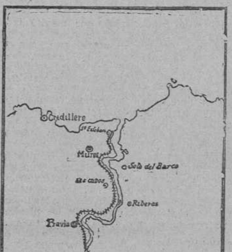
Copia hecha sobre el Mapa Militar Itinerario de España, formado por el Cuerpo de Estado Mayor del Ejército en 1920, en la parte correspondiente al croquis publicado en EL DEBATE del 25 de noviembre de 1926.
