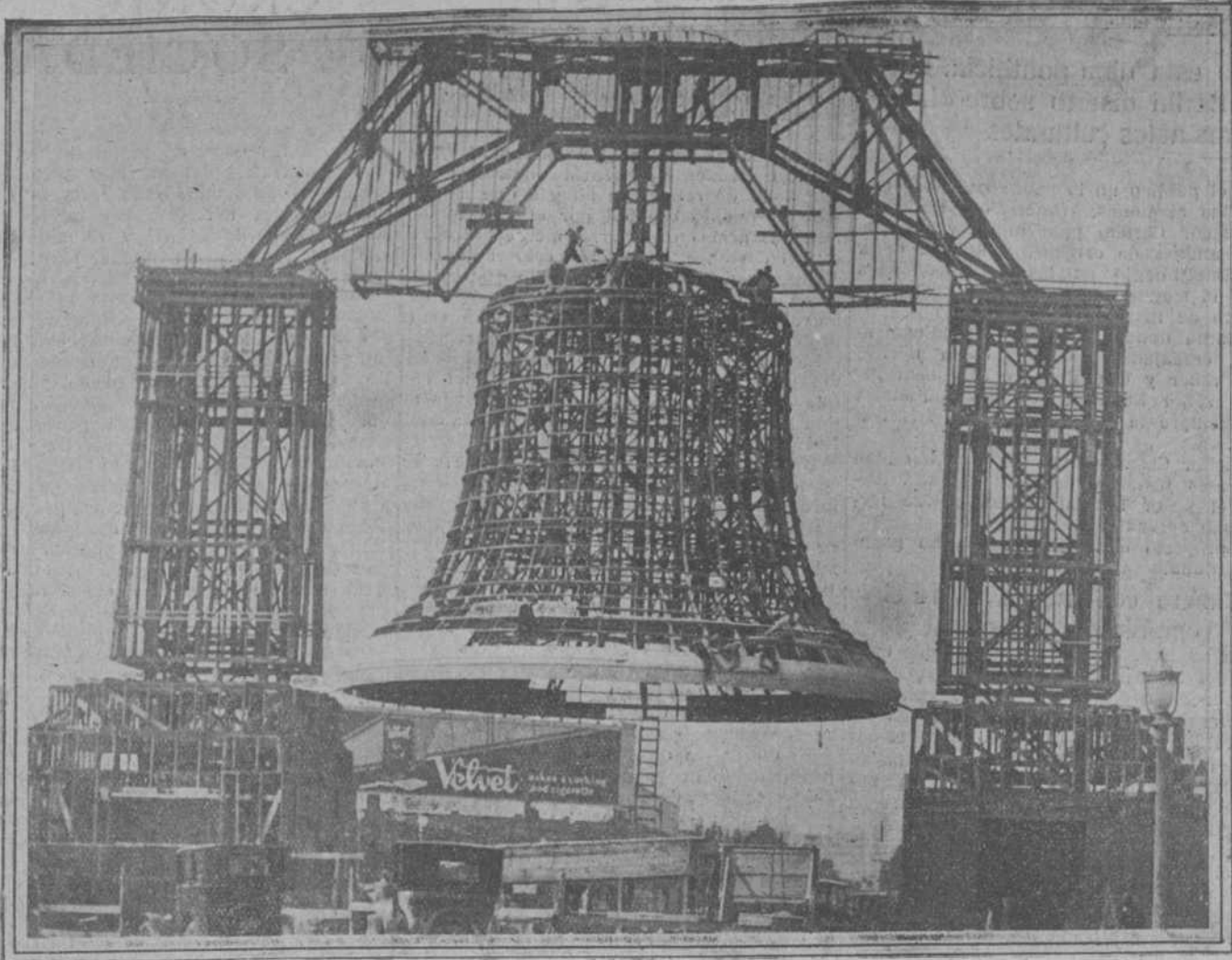
La gran campana de la Libertad, que se está construyendo para la puerta del estrado de la Exposición de Filadelfia. Pesará 82 toneladas y tiene 70 pies de altura y 50 de ancho. Por las noches estará iluminada con 26.000 bombillas. (Fot. Vidal.)
