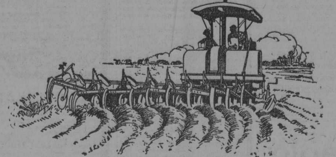
Máquina "Tracklayer" 75 H. P. rompiendo tierra con 10 arados en el Contr al "Portugalete"
