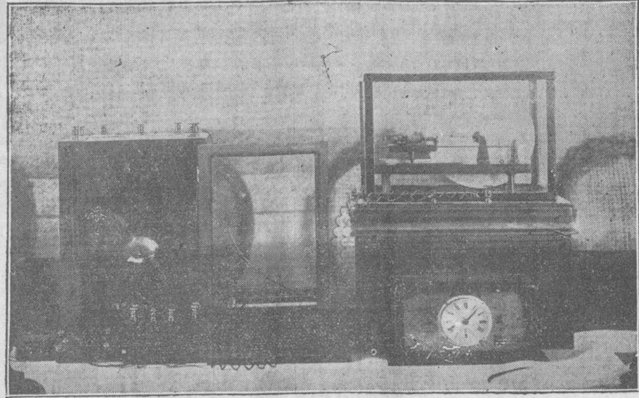
CIENCIA METEOROLOGICA. Aparato registrador de descargas eléctricas, que funciona en el Observatorio del Colegio Nuestra Señora de Montserrat de los padres Jesuitas en Cienfuegos.
