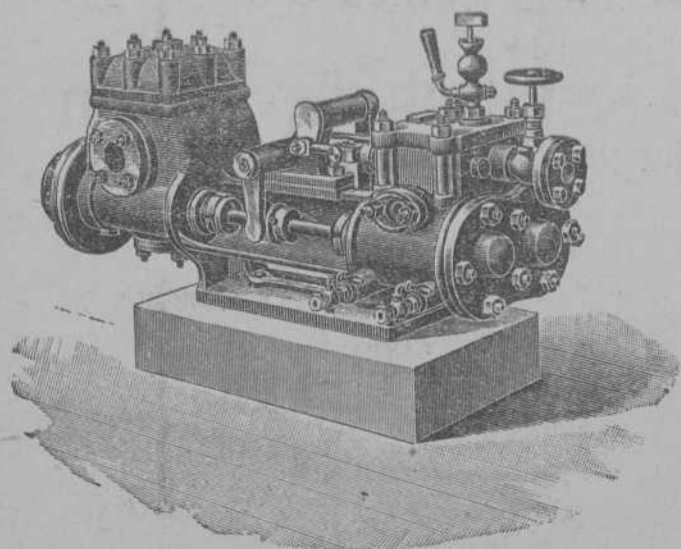
Bomba de vapor «DUPLEX»
