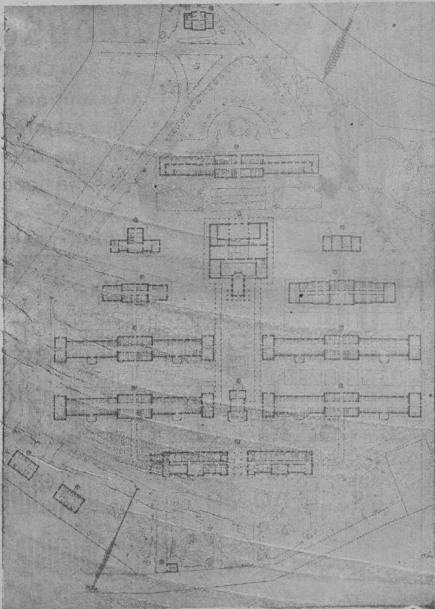
ANTEPROYECTO DEL HOSPITAL PROXIMO A CONSTRUIRSE EN SANTANDER, OBRA DE LOS ARQUITECTOS SEÑORES MARTINEZ DEL VALLE Y URCOLA.
