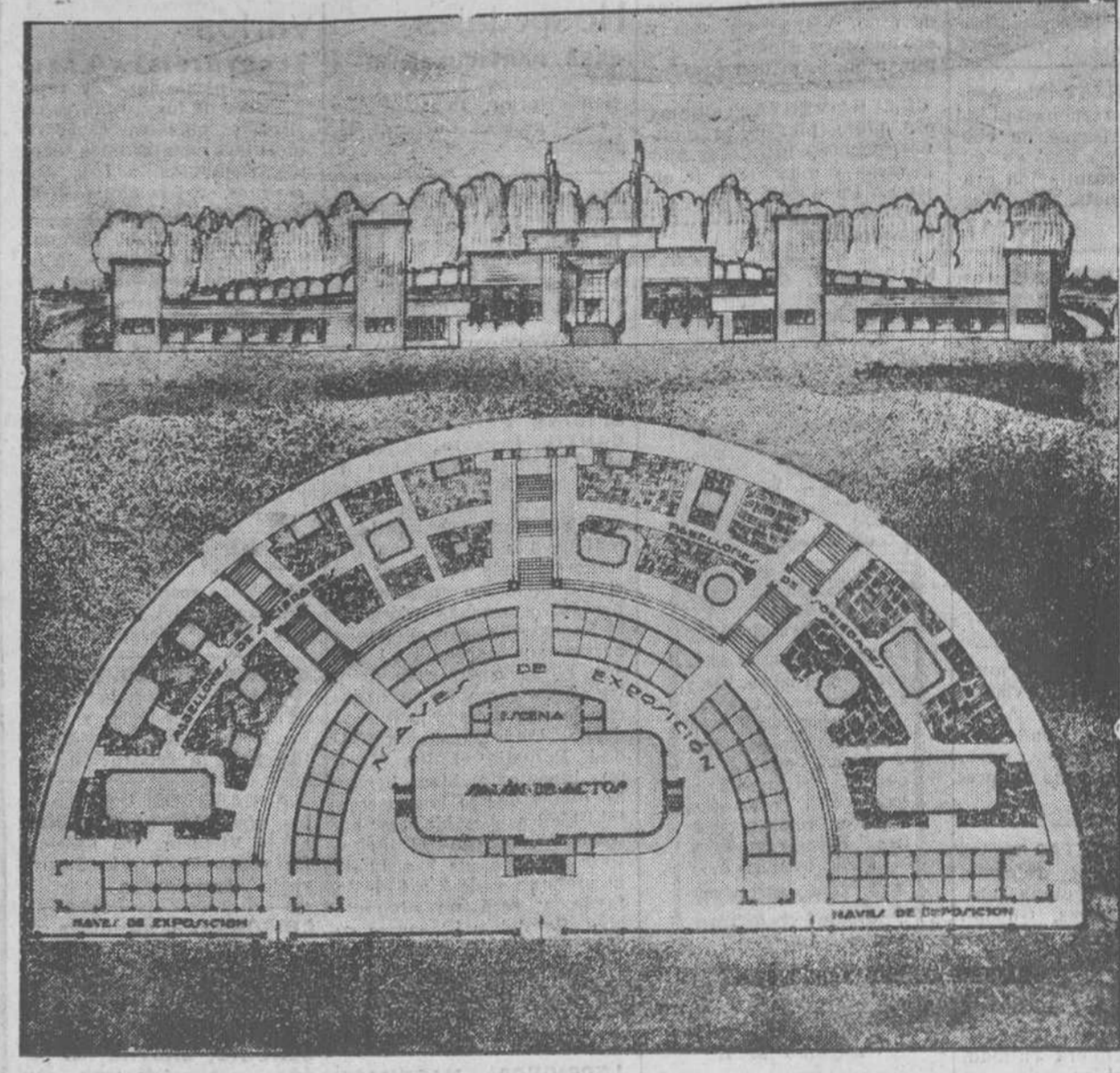
He aquí, en unos trazos de pluma experta, lo que pudiéramos llamar la osamenta de la proyectada FERIA DE MUESTRAS. Arriba, una perspectiva de la instalación en su aspecto exterior; abajo, descripción gráfica de los distintos departamentos.
