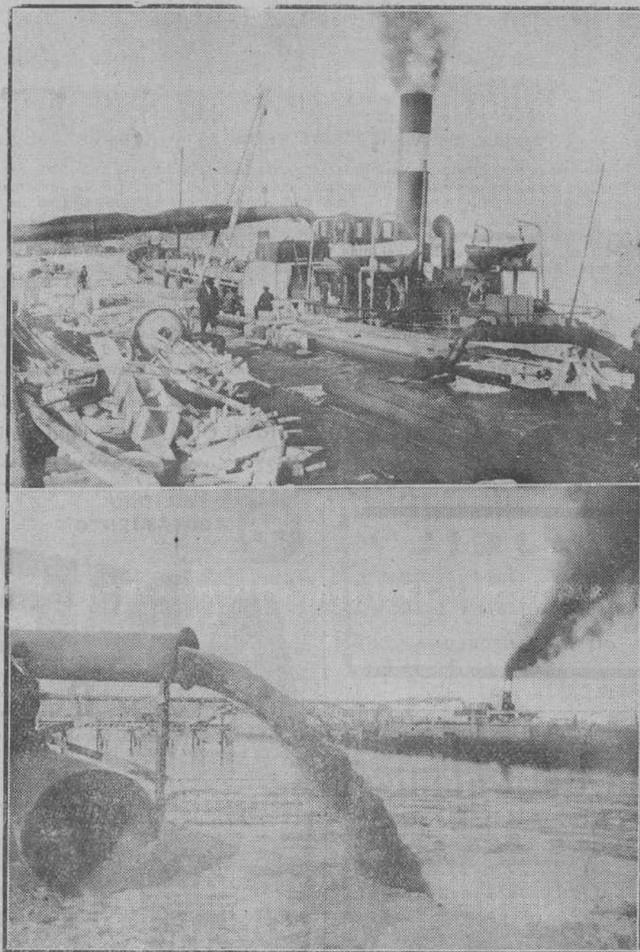
LAS OBRAS DE LOS NUEVOS MUELLES. —La potente bomba de la draga «Cantabria», atracada al nuevo muelle de hormigón, envía, a través de una tubería de más de cien metros de extensión, la arena que extrae de la bahía. Abajo: La salida del gran tubo, que escupe diariamente más de tres mil toneladas de arena, constituyendo el firme que lentamente va empujando al mar fuera de la línea de los muelles recién construidos. (Foto Alejandro.)
