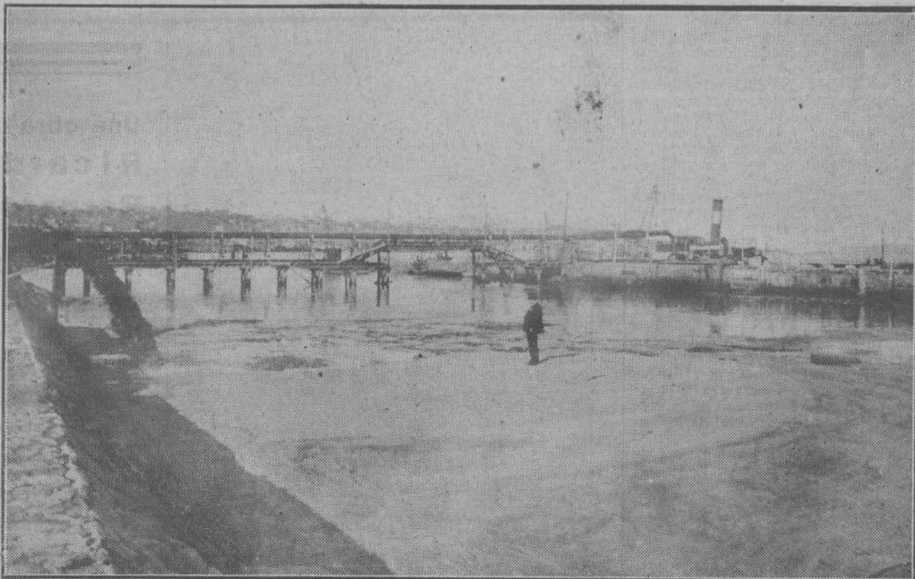
LAS OBRAS DE LOS NUEVOS MUELLES.—Santander, en su lucha de conquista contra el mar, lucha iniciada hace siglos, gana terreno diariamente. Esta foto nos demuestra cómo la ciudad extiende sus dominios «construyendo», con la ayuda de la draga «Cantabria», la playa que, antes de muchos días, ha de unir los dos muros—el viejo de la escollera y el moderno de los muelles—para convertirse en una magnífica avenida frente al Depósito Franco. (Foto Alejandro.)
