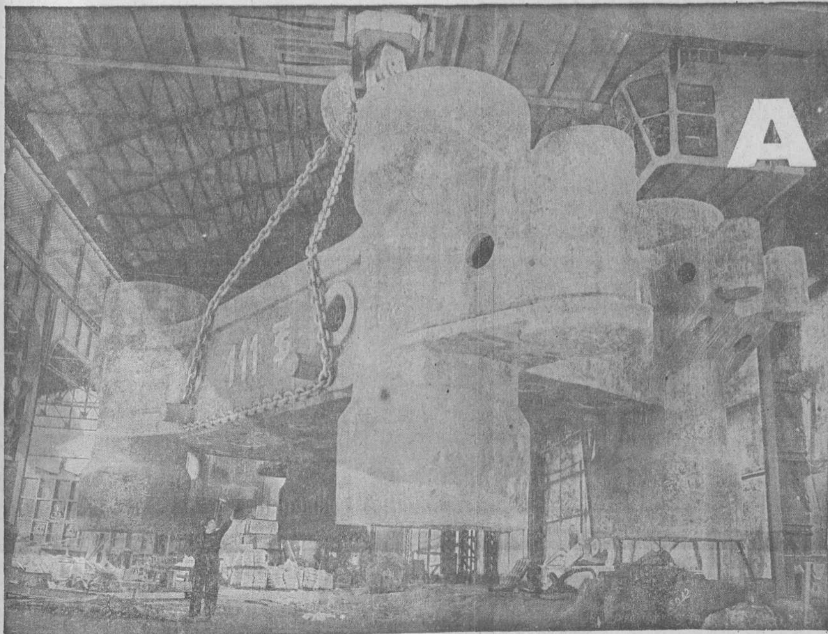
PIEZA DE ACERO MOLDEADO DE 111 TM. PARA PRENSA DE 6.300/7.500 TM. FUNDIDA EN NUESTROS PROPIOS TALLERES
