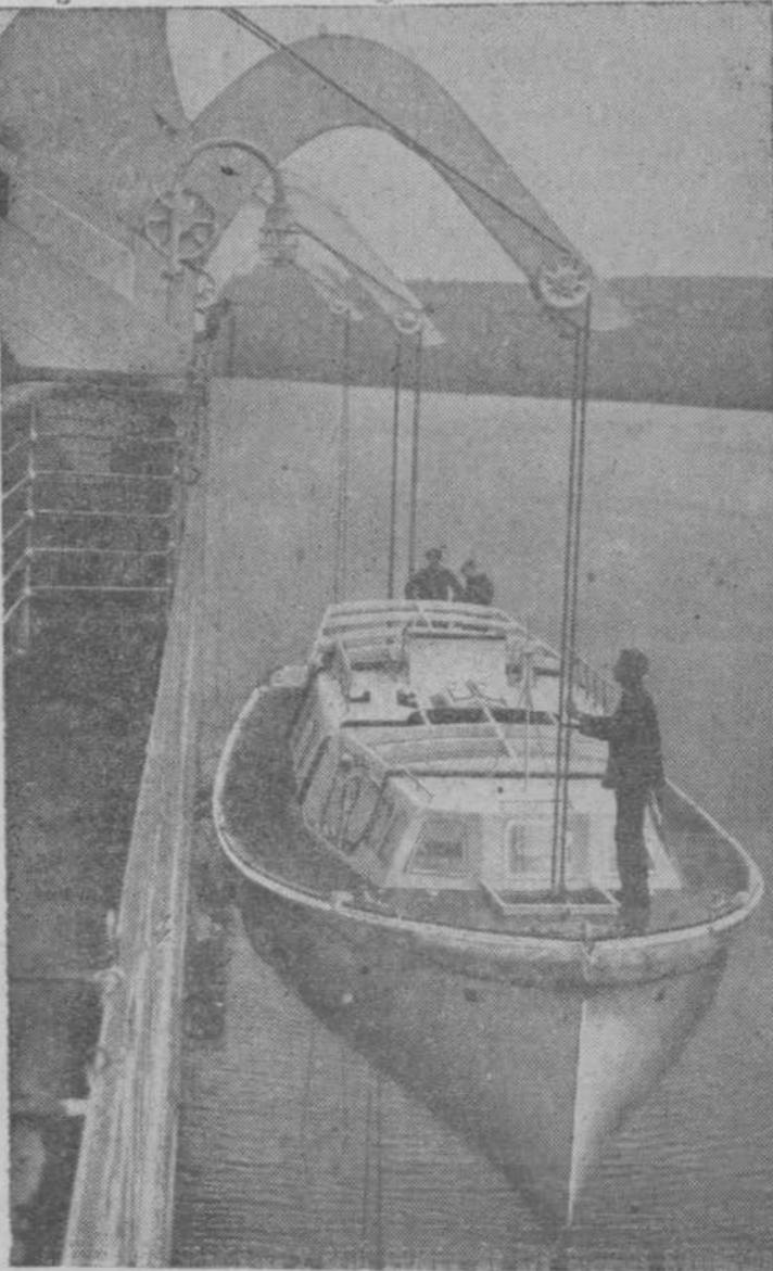
Pruebas del funcionamiento de un bote de salvamento. Puede admitir 60 pasajeros y está dotado de los últimos adelantos
