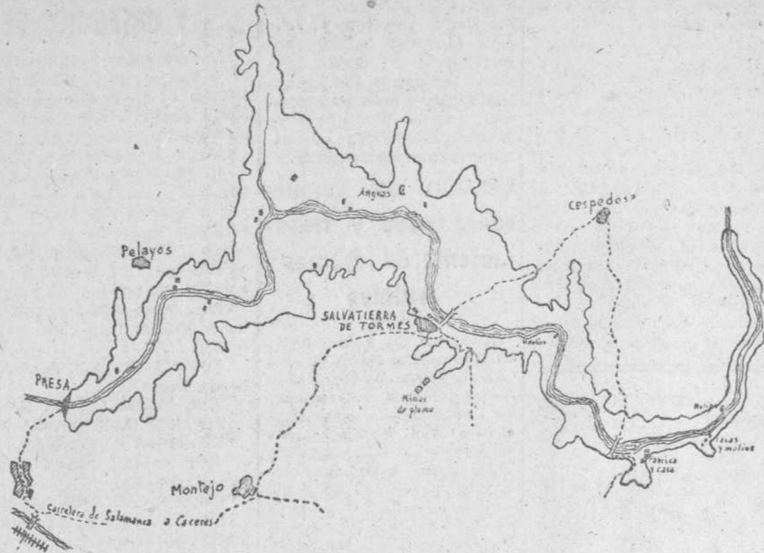
Esquema del embalse del pantano de Santa Teresa. En él, a ambos lados del curso del Tormes, y a partir de la presa, se extiende una línea continua que marca los límites del embalse o terreno inundado. Las líneas interrumpidas significan caminos o carreteras. El plano está hecho a una escala aproximada de 1:120.000, con la que el lector puede imaginarse las dimensiones, que en Salvatierra serán de más de 2 kilómetros de anchura
