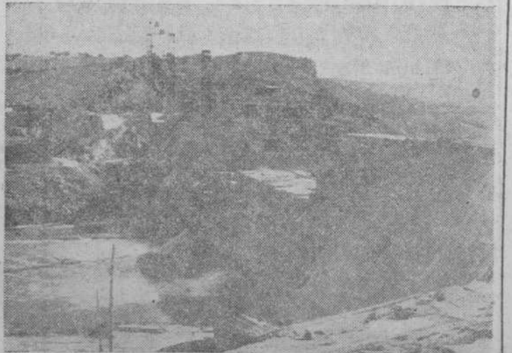
Vista de la presa, por su parte de aguas abajo, y en primer término, la parte de talud ya terminada y las entradas a las galerías interiores. (Foto Guzmán Gombau.)
