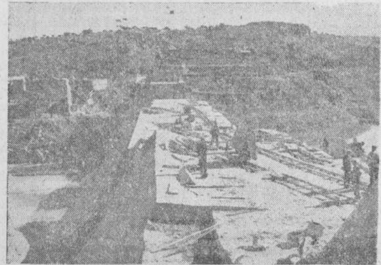
La presa, vista desde la parte superior. Al fondo, la torreta levantada en el punto de mayor altura, y a la izquierda los paramentos concluidos. (Foto Guzmán Gombau.)
