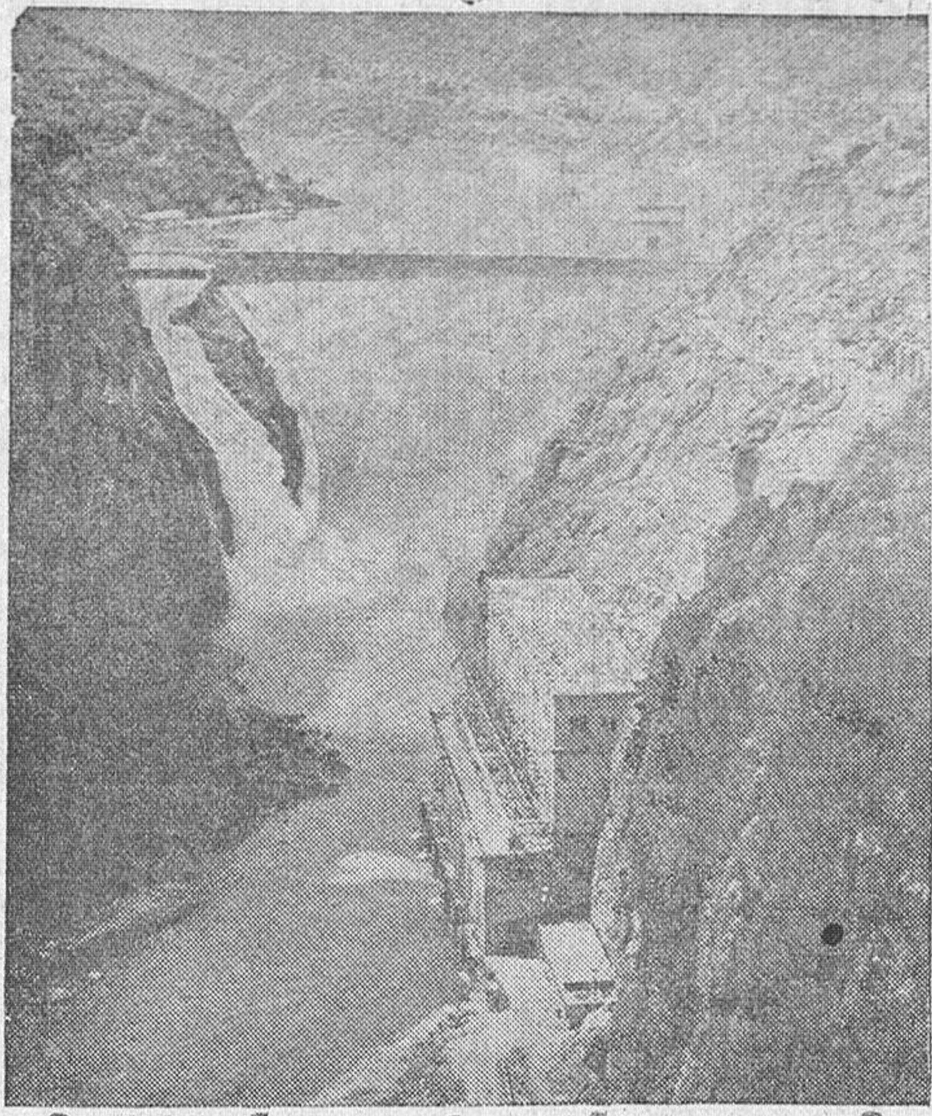
Central y presa de Camarasa (Lérida). La altura de ésta es de 92 metros y la potencia instalada, es de 88.000 C. V.
