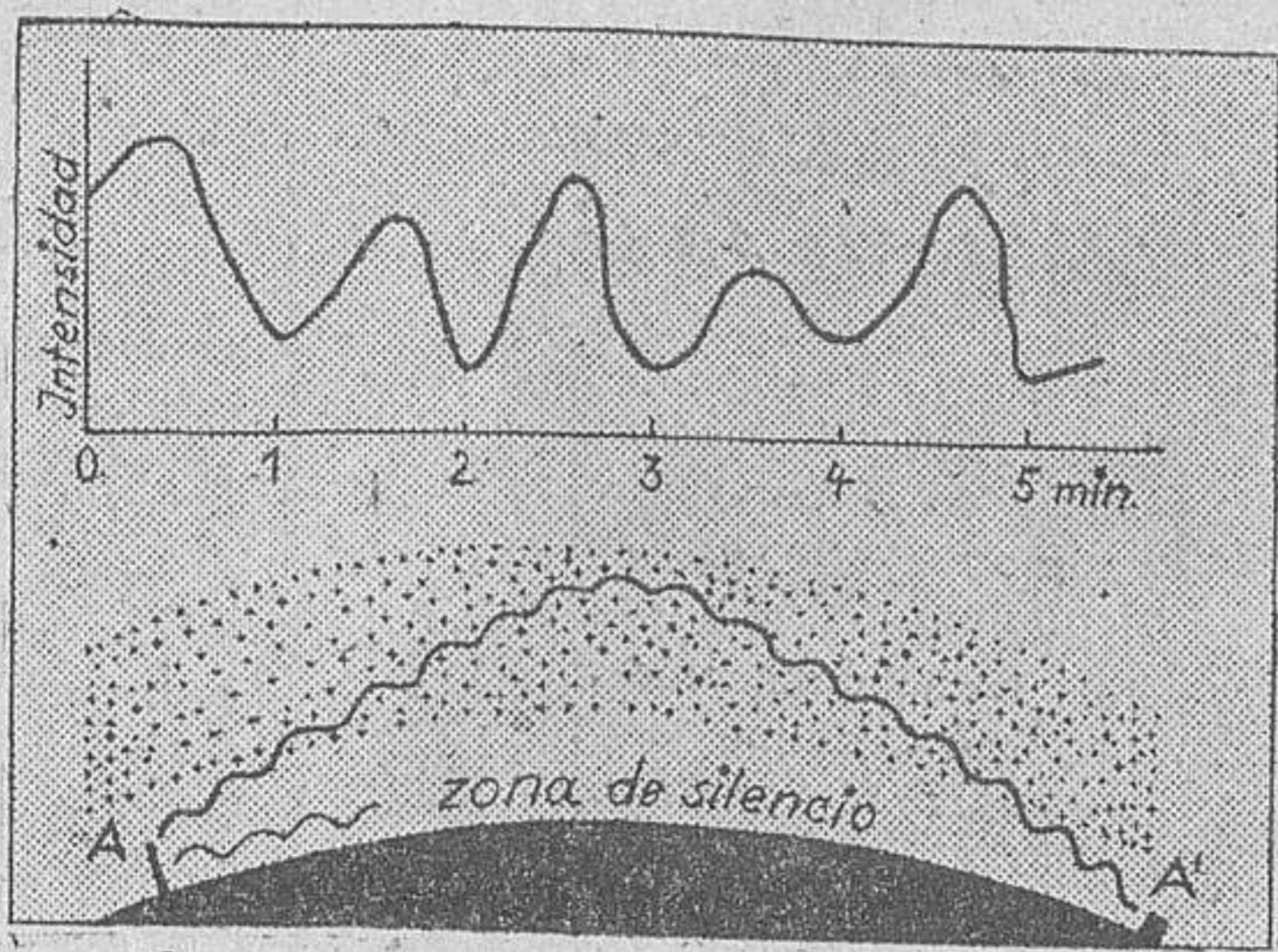
Curva de periodicidad del fading
