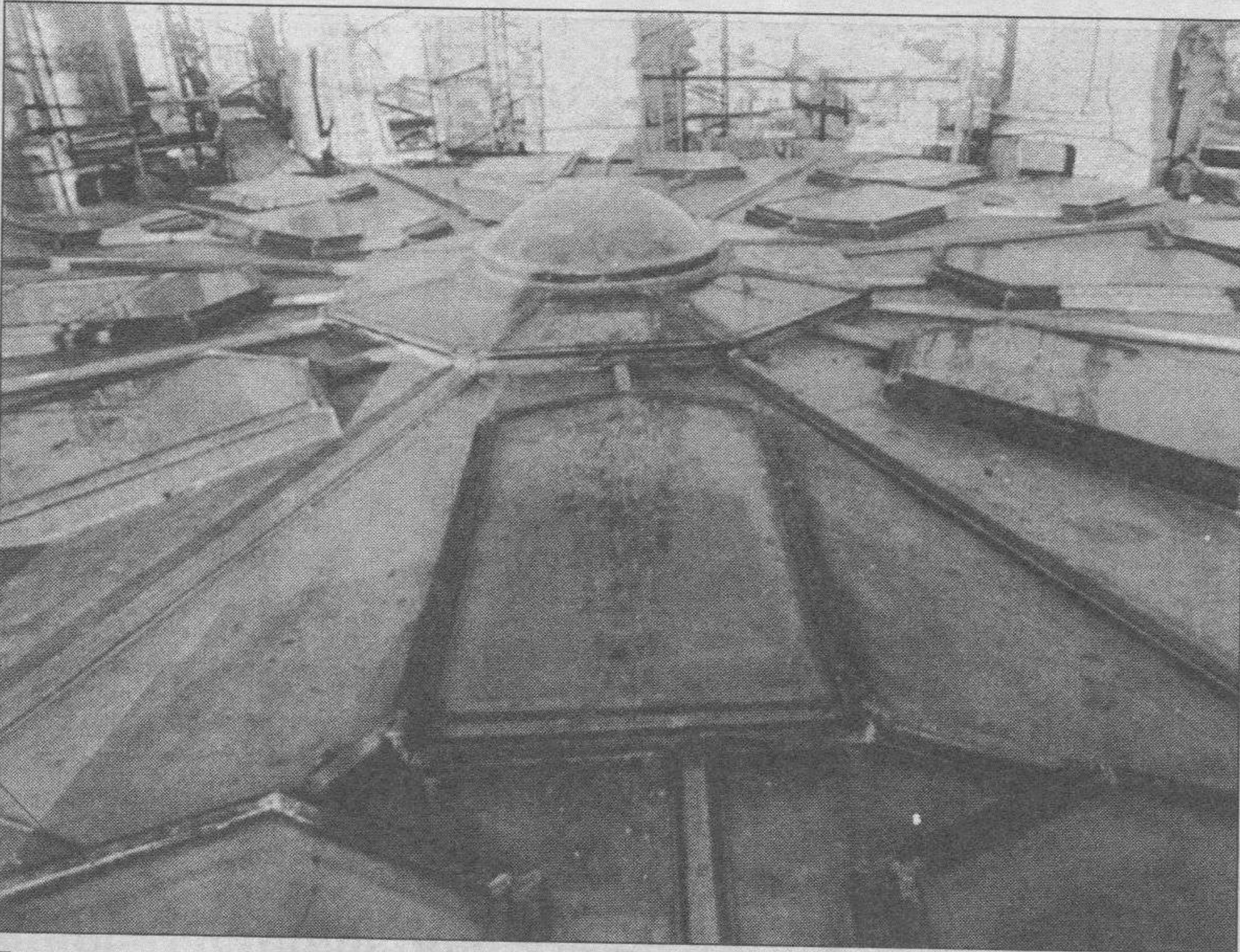
Estructura exterior del lucernario del Crucero.
