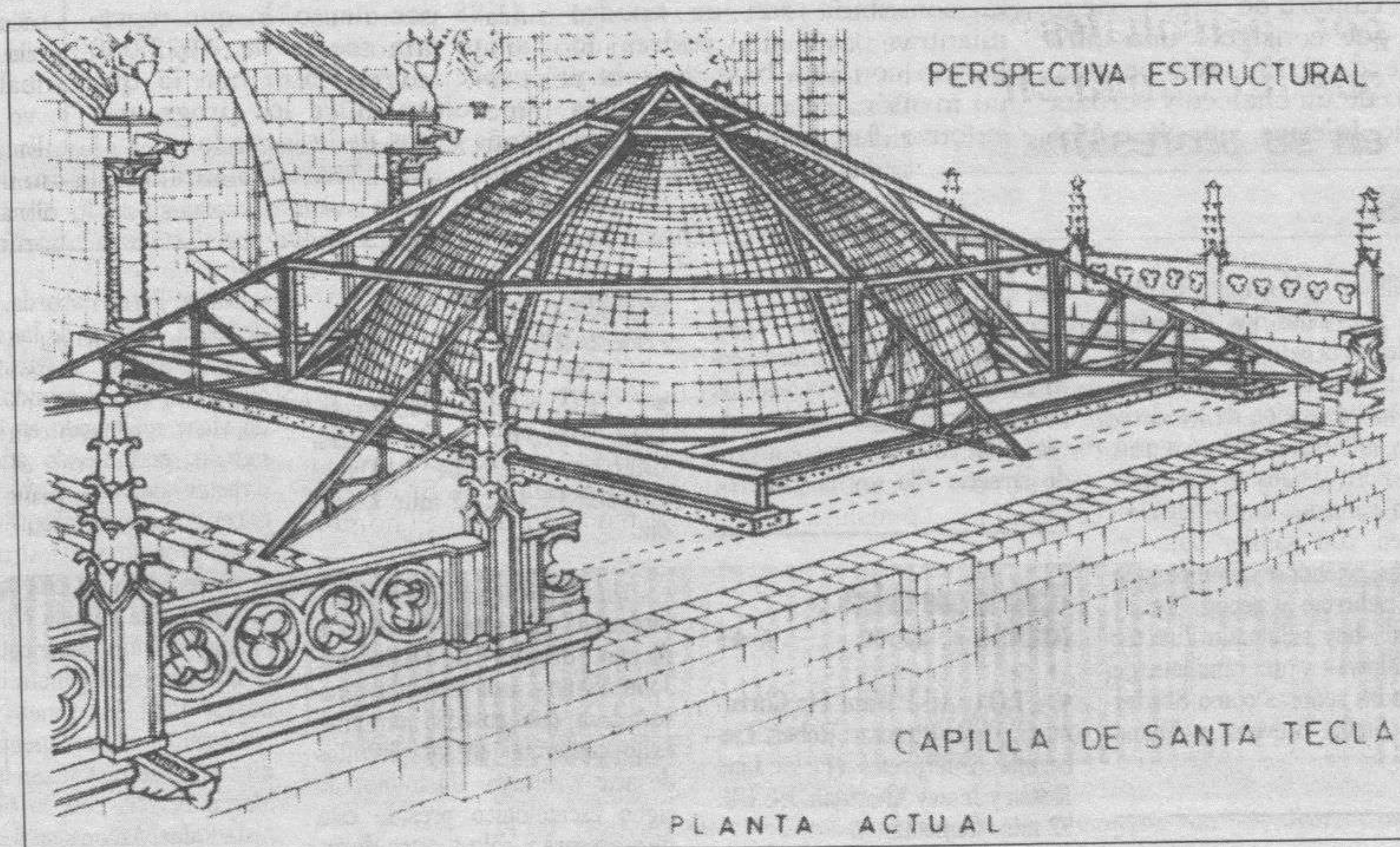
La estructura de la nueva cubierta de Santa Tecla.
