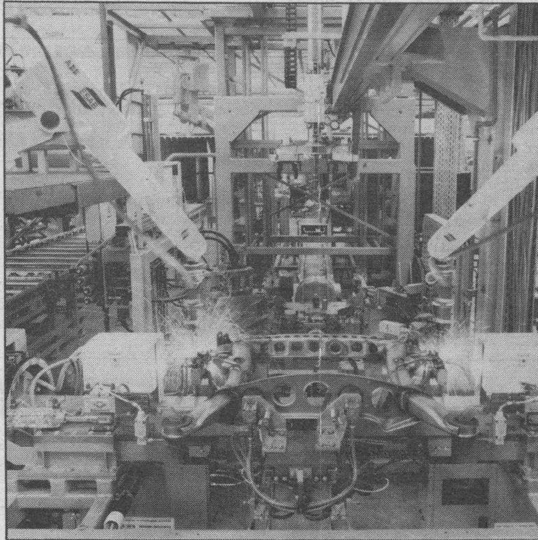
Fase del proceso de fabricación de brazo de suspensión.
