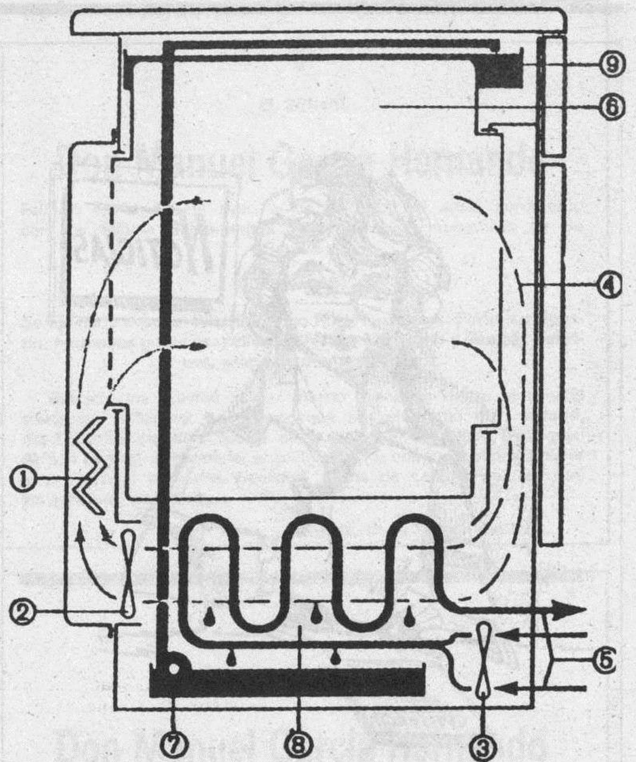
La secadora: 1: Resistencia. 2: Ventilador de aire caliente húmedo. 3: Ventilador de aire frío. 4: Aire caliente. 5: Aire frío. 6: Tambor. 7: Bomba de agua de condensación.
