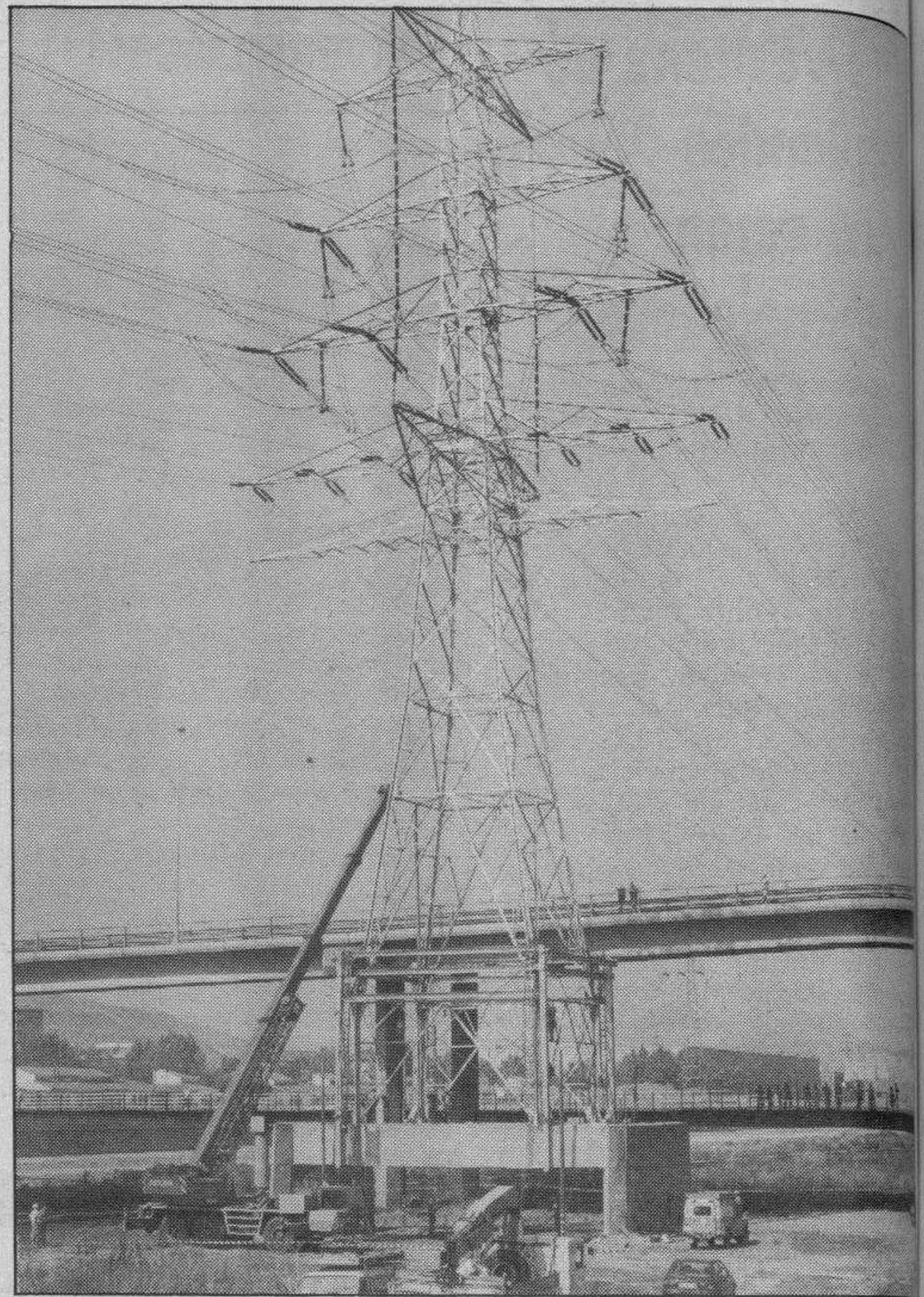
Obras en una columna de la red de distribución.
