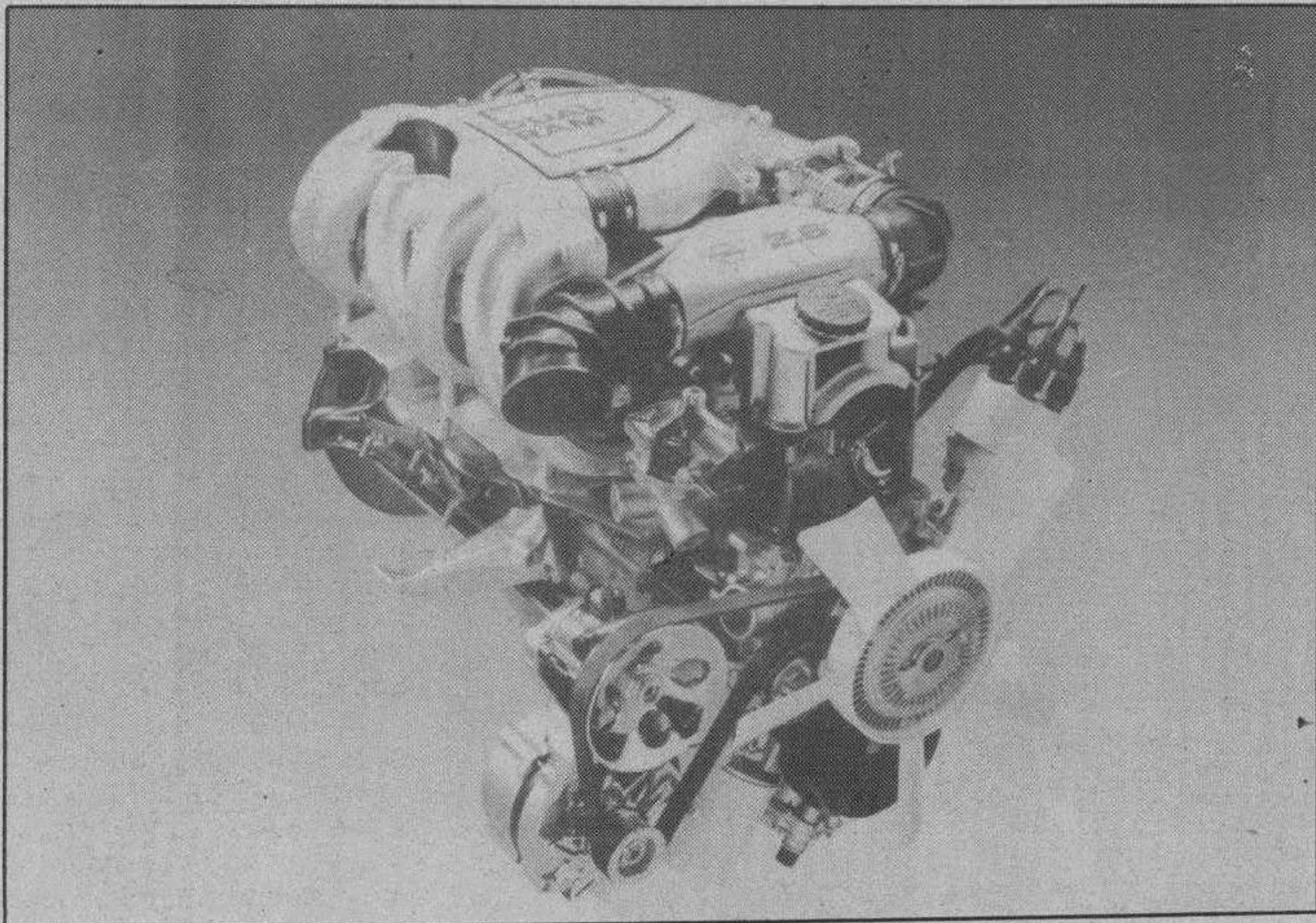
El nuevo motor dispone de 2.594 cc., 6 cilindros y 150 CV
