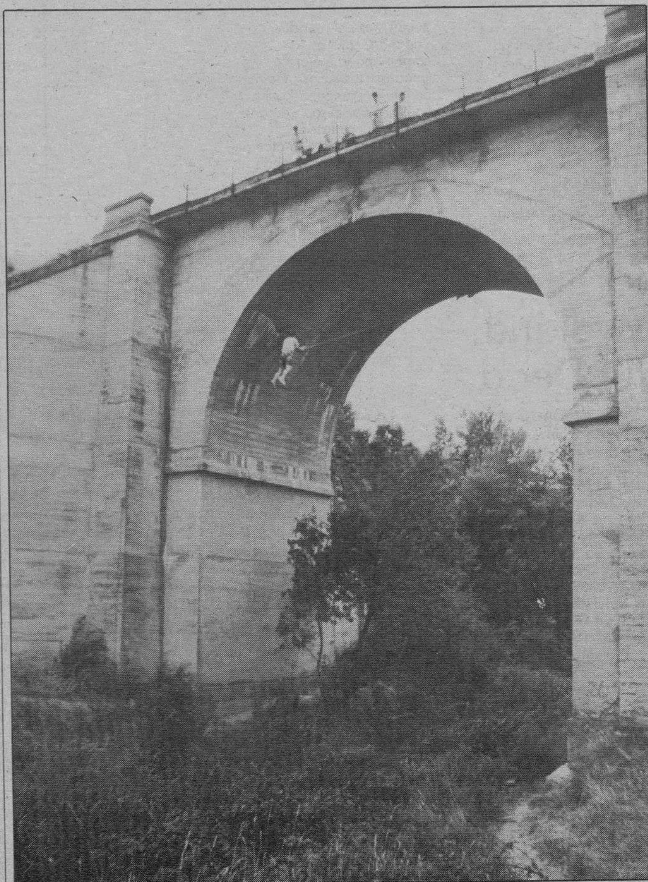
El puente, por el cual pasa el ferrocarril Madrid-Burgos, tiene una luz de 25 metros.
