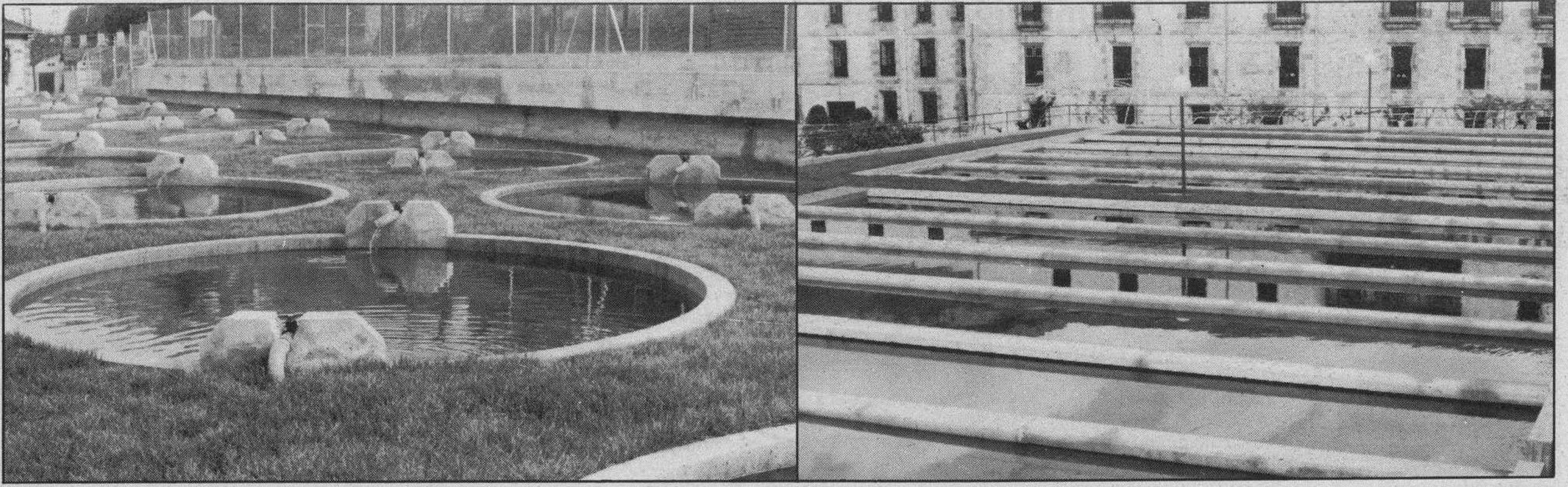
Estanques circulares rectangulares de la piscifactoría de la Diputación en Oña.
