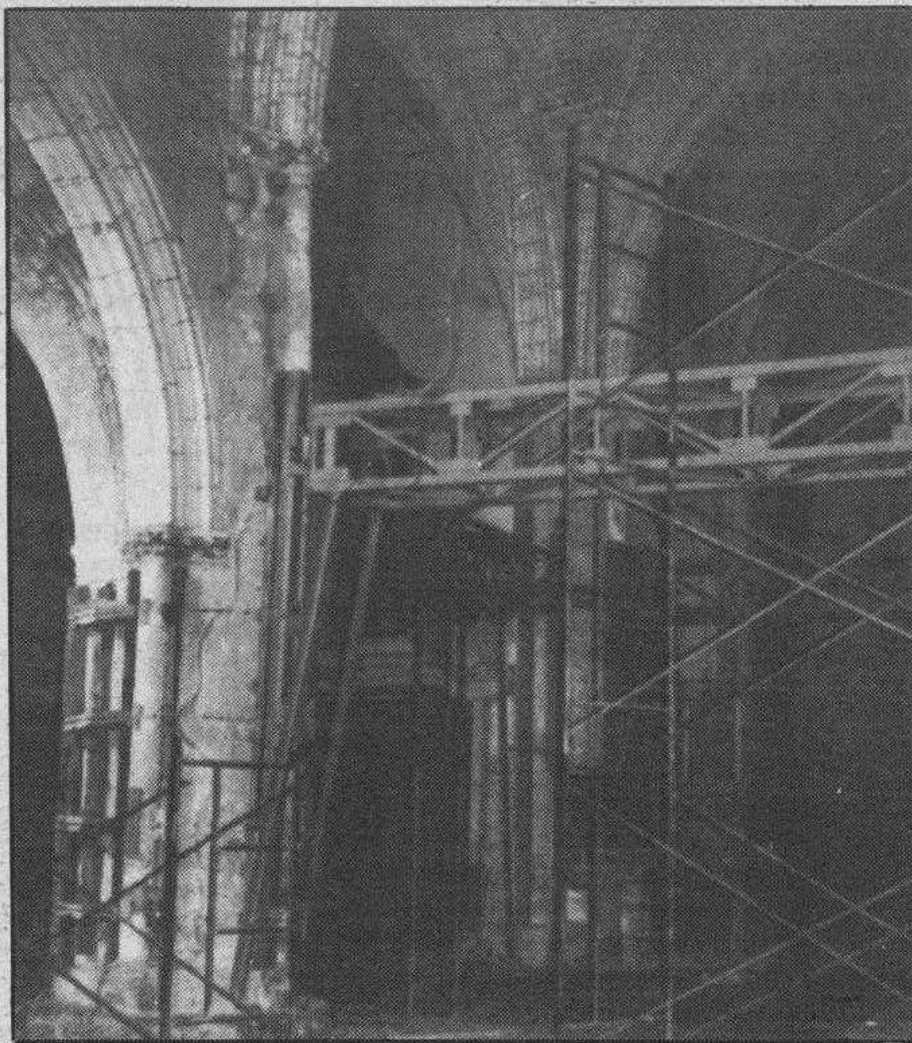
Vista interior con estructuras metálicas apuntalando algunas columnas.
