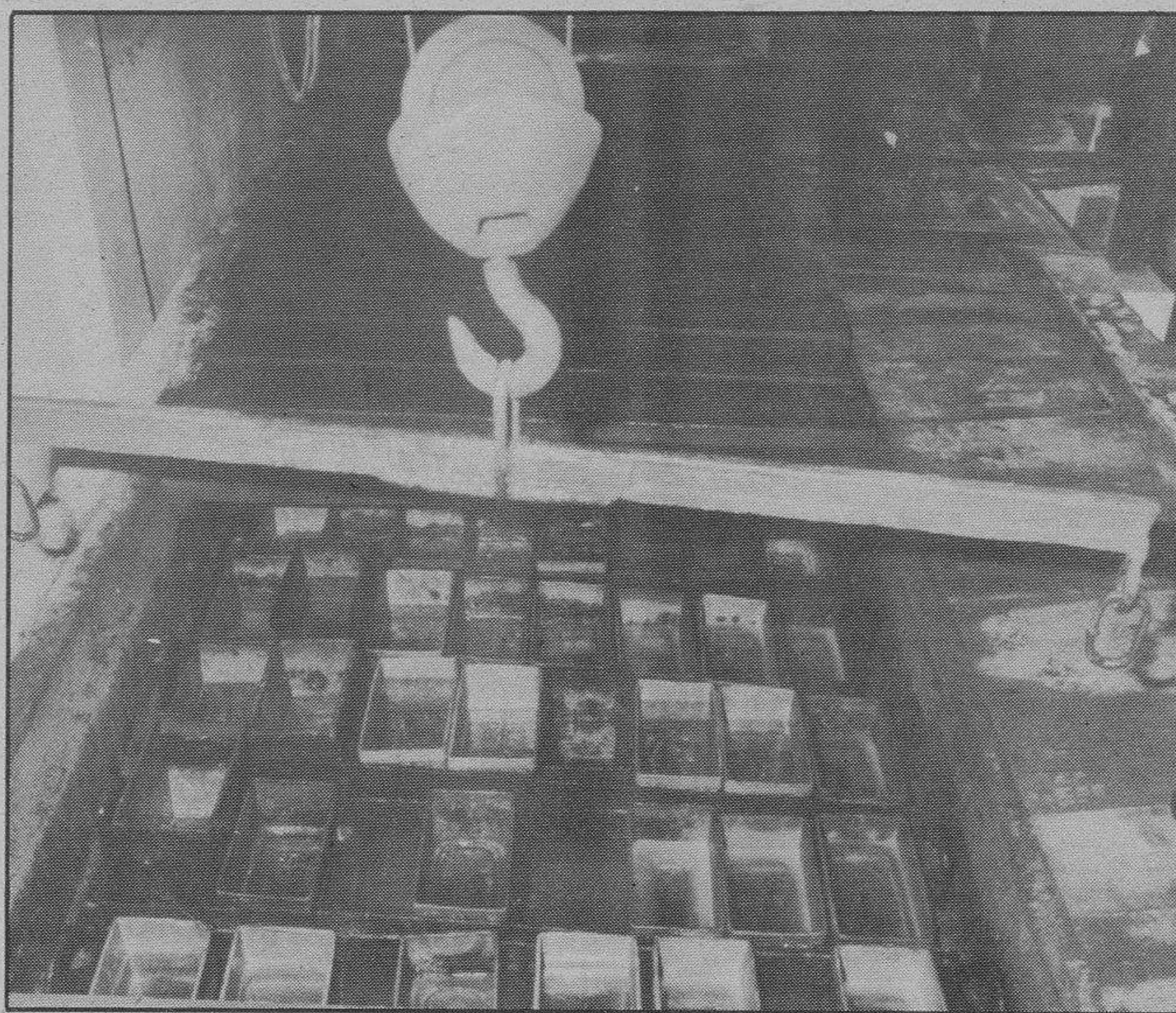
El agua se convierte en hielo en el interior de unos moldes, que se introducen en la balsa que tiene un preparado de «salmuera» en el fondo.
