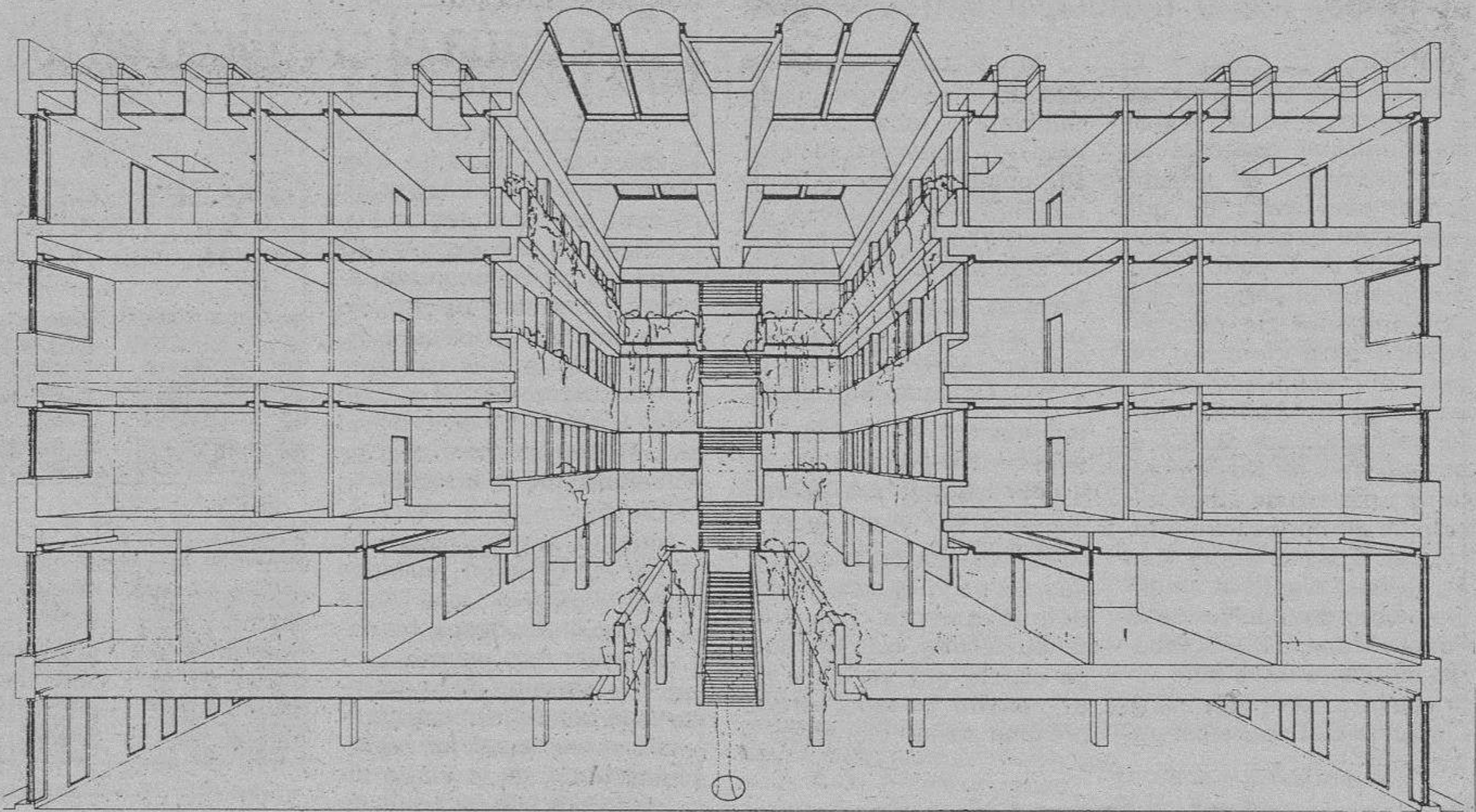
Perspectiva cónica. Sección transversal del proyecto.
