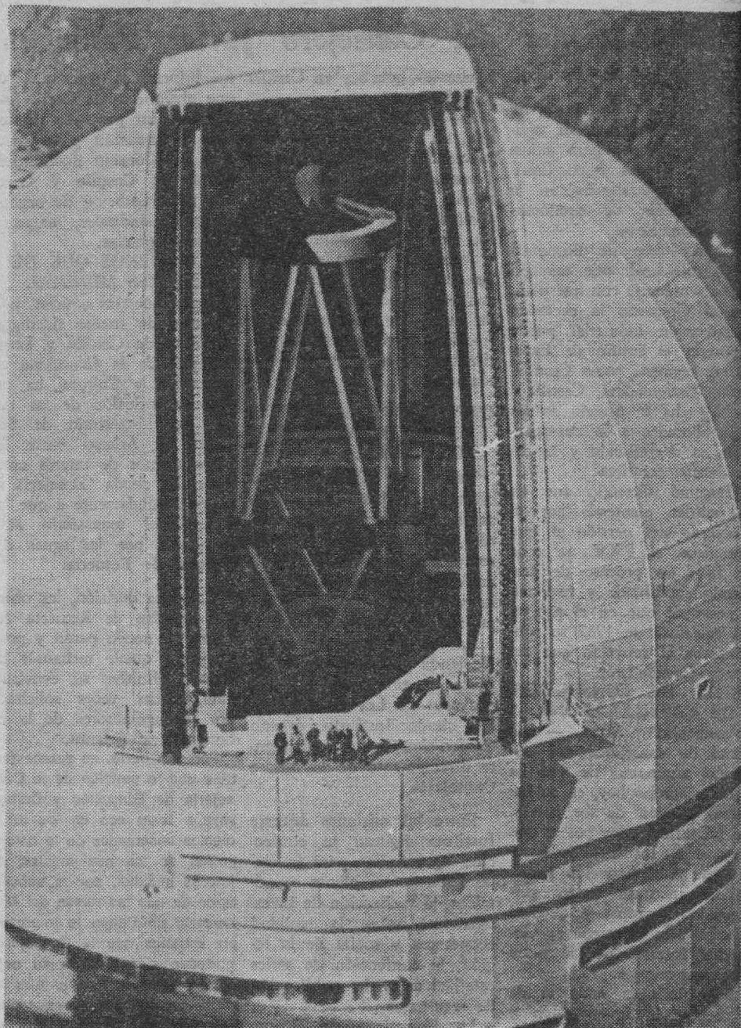
TELESCOPIO ACIMUTAL CON CRISTAL DE SEIS METROS DE DIAMETRO
