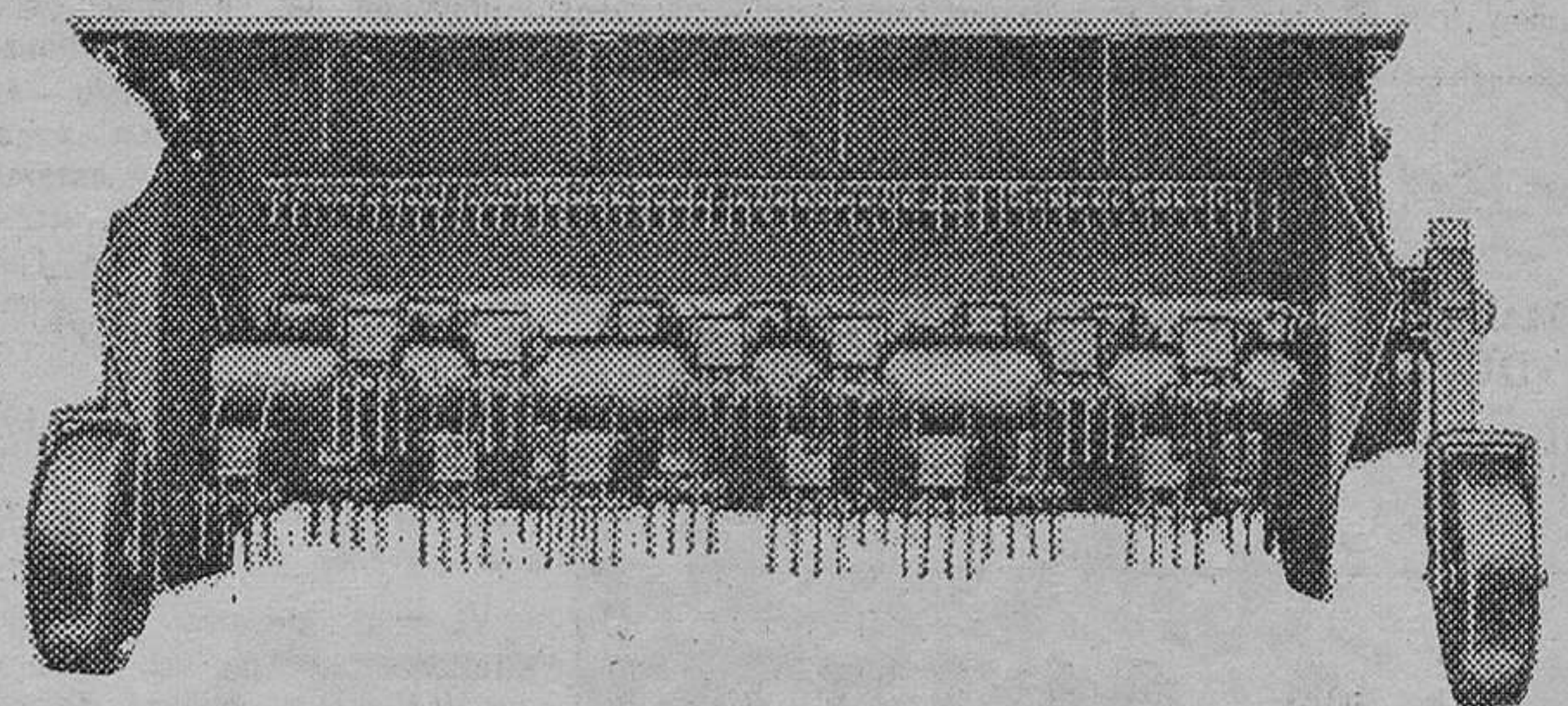
DESBROZADORA DE PAJA —JF— DE 1,60 Y 2,10 CORTE
