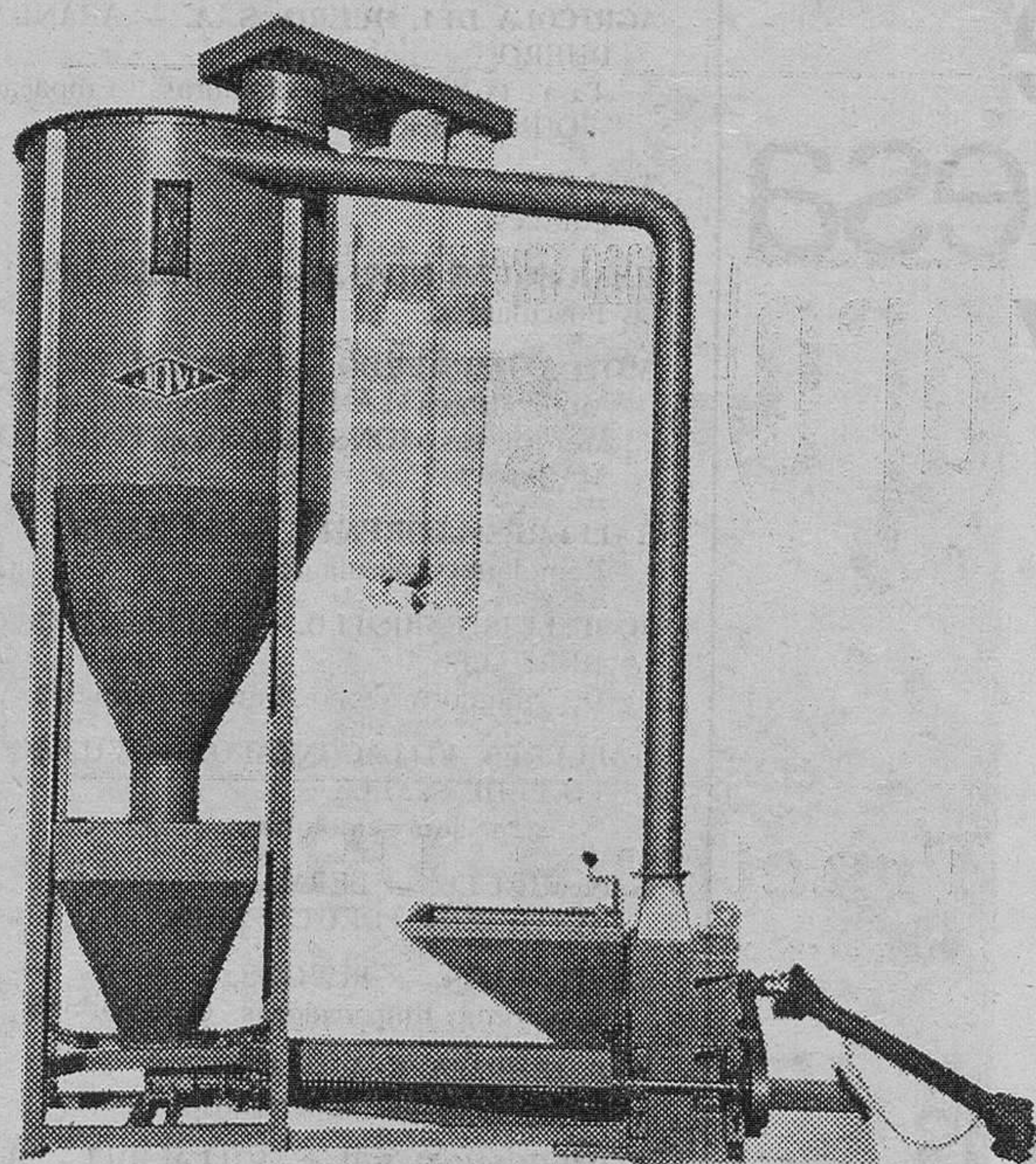
Conjunto de molino y mezcladora vertical
