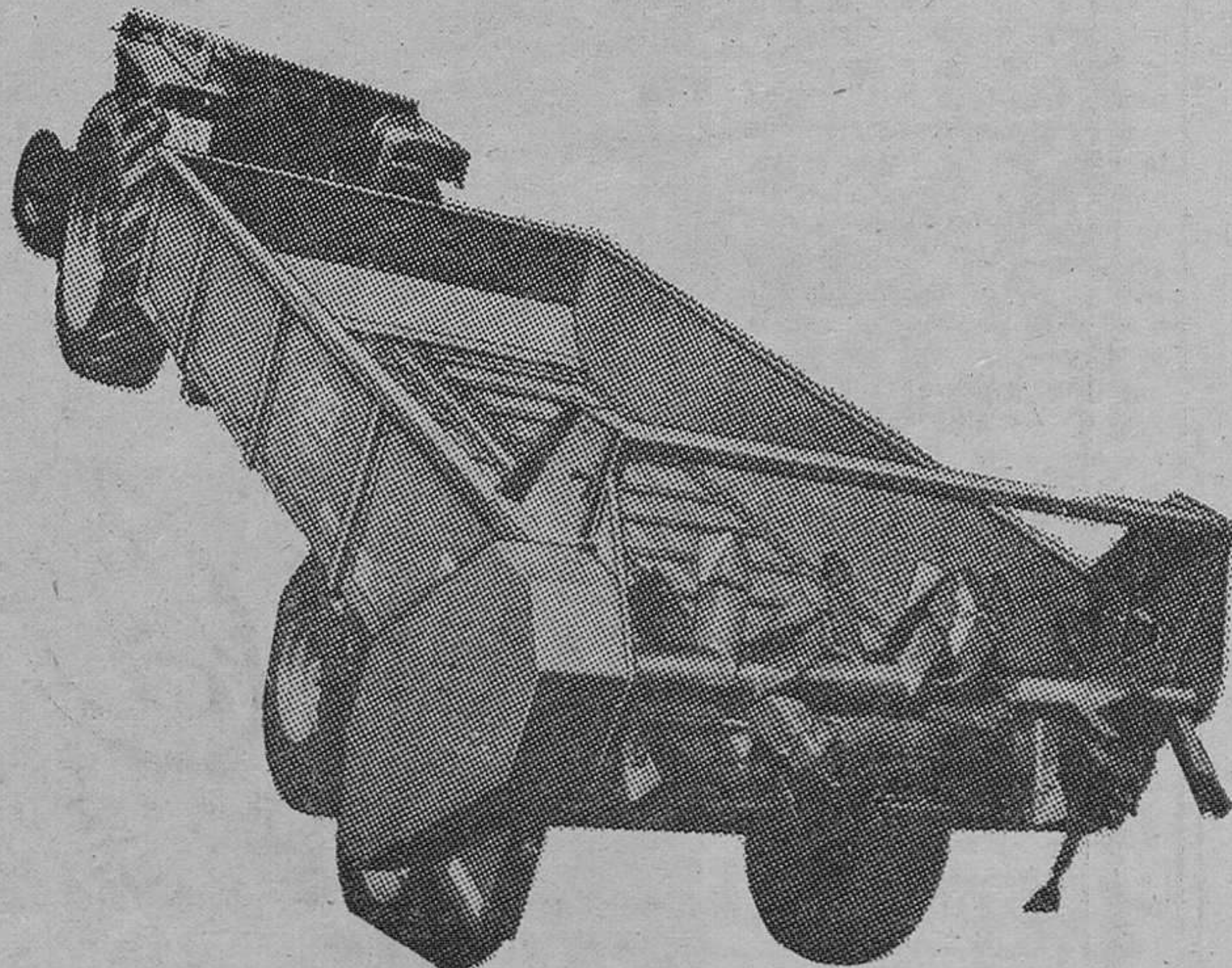
SUPERTRANSPORTE TIPO «ST 90» DE 9.000 KILOS
