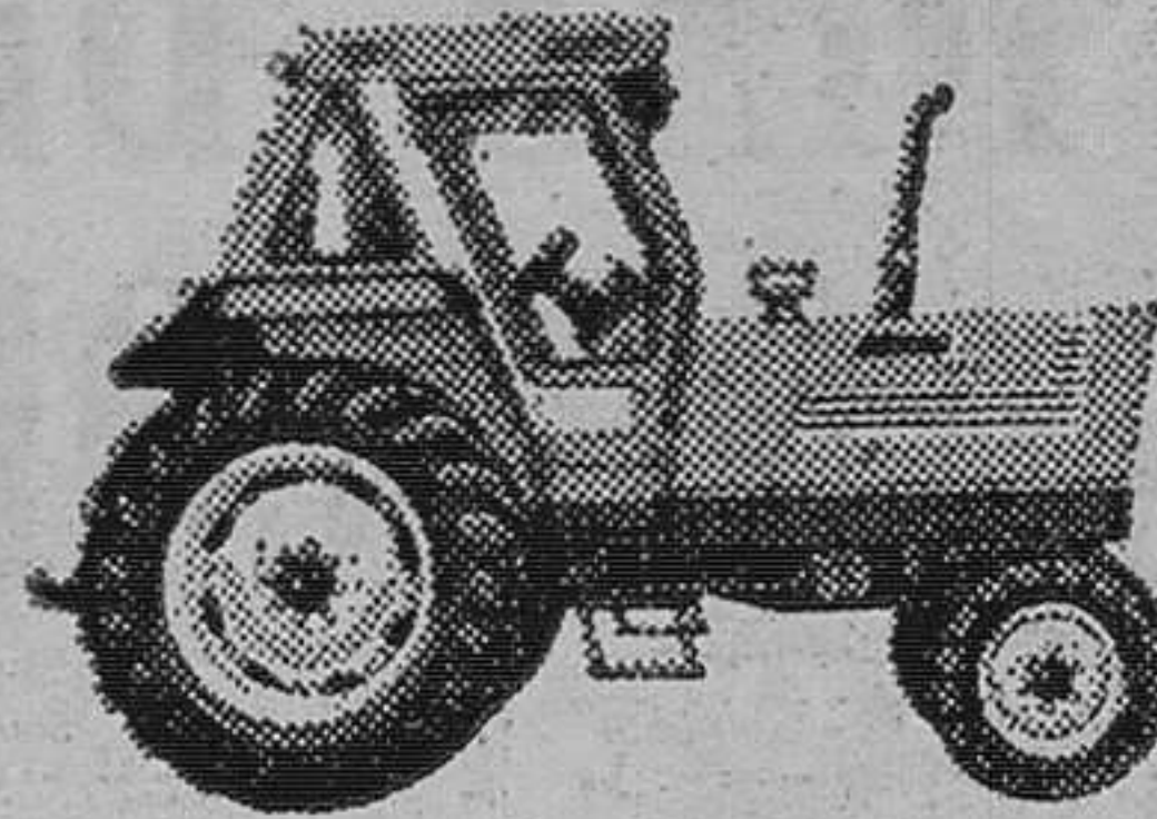
1380 135 CV 5450 Kg
