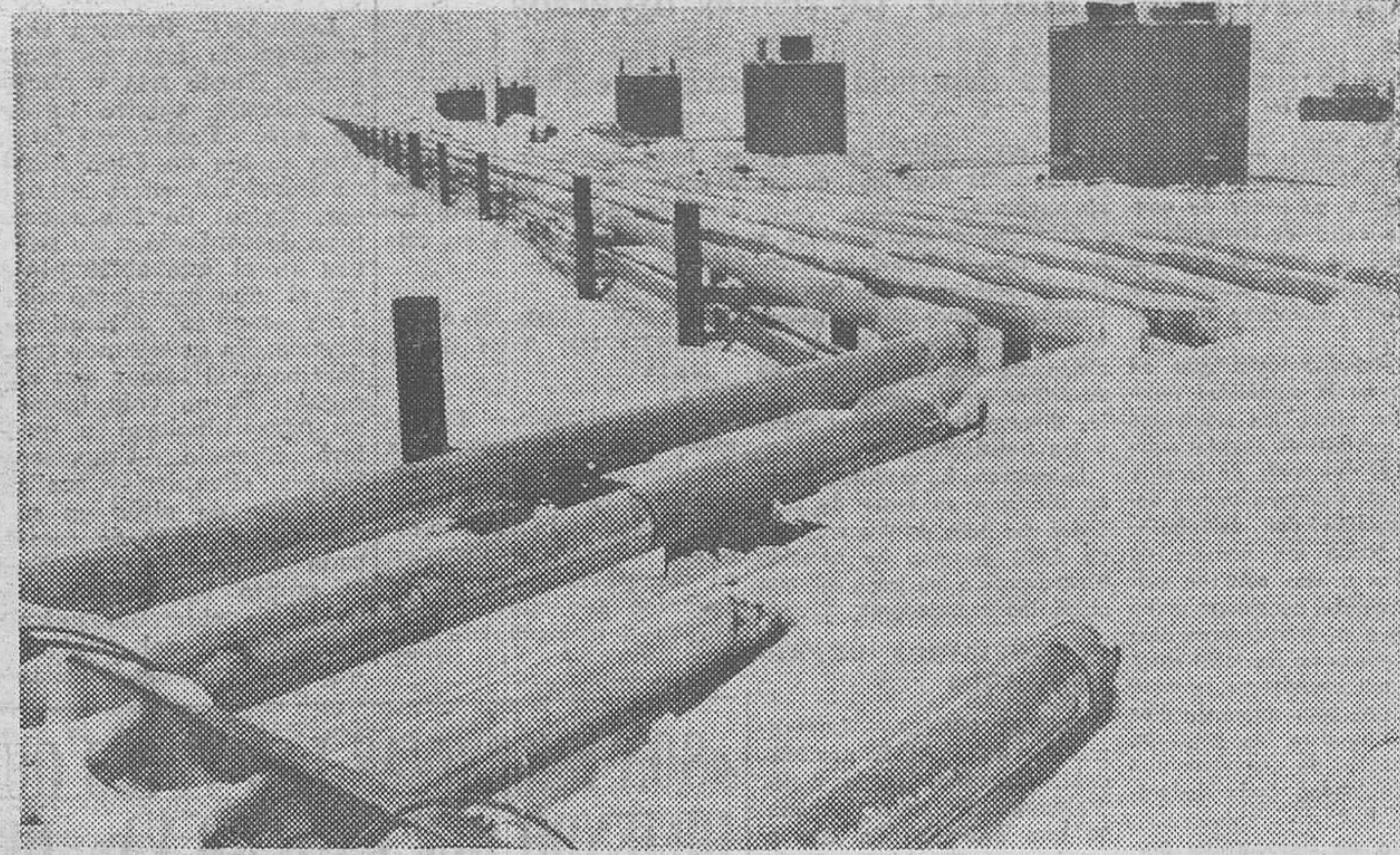
Los conductos que llevan el petróleo desde Prudhoe Bay hasta el centro número uno. Las instalaciones de control están protegidas de los cambios atmosféricos mediante unas construcciones metálicas.—(Foto EFE).
