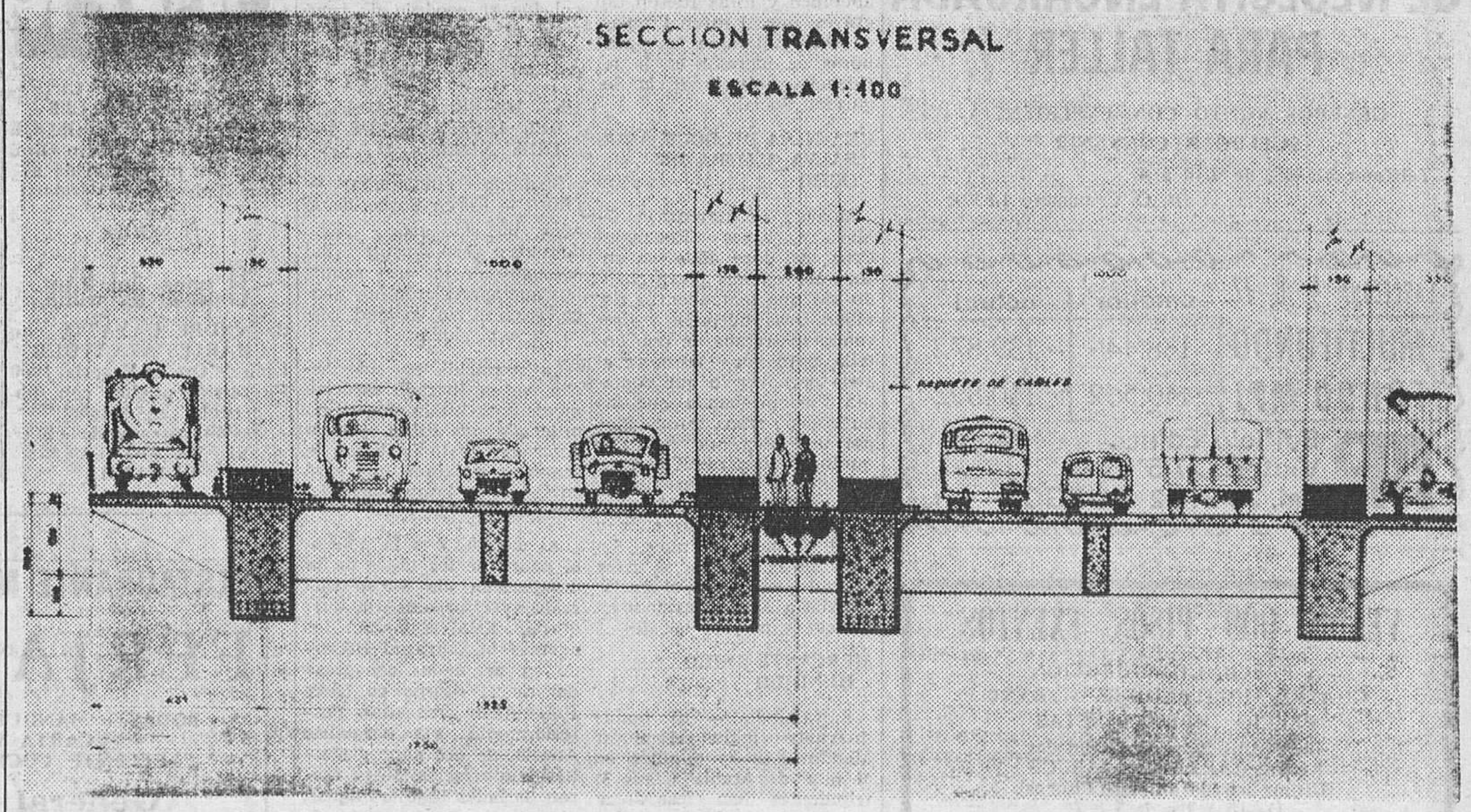
Sección transversal del proyecto de puente sobre el Estrecho de Gibraltar, del ingeniero señor Peña Boeuf. — (Foto LOGOS).
