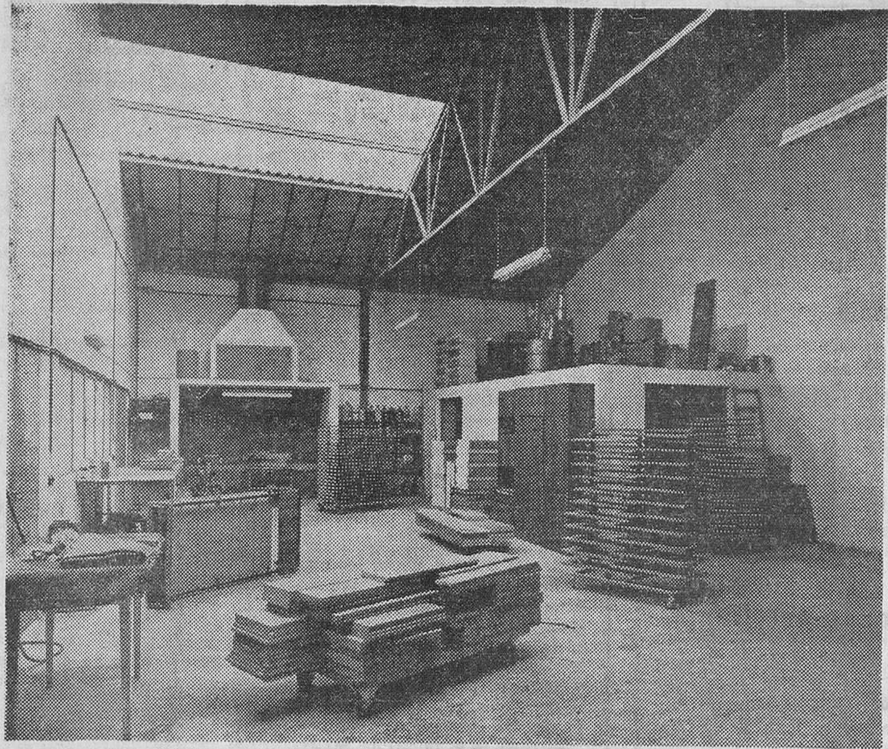
(SECCION DE BARNIZADO Y HORNO DE SECAJE DE NUESTRA FABRICA EN CASTANAEROS)
