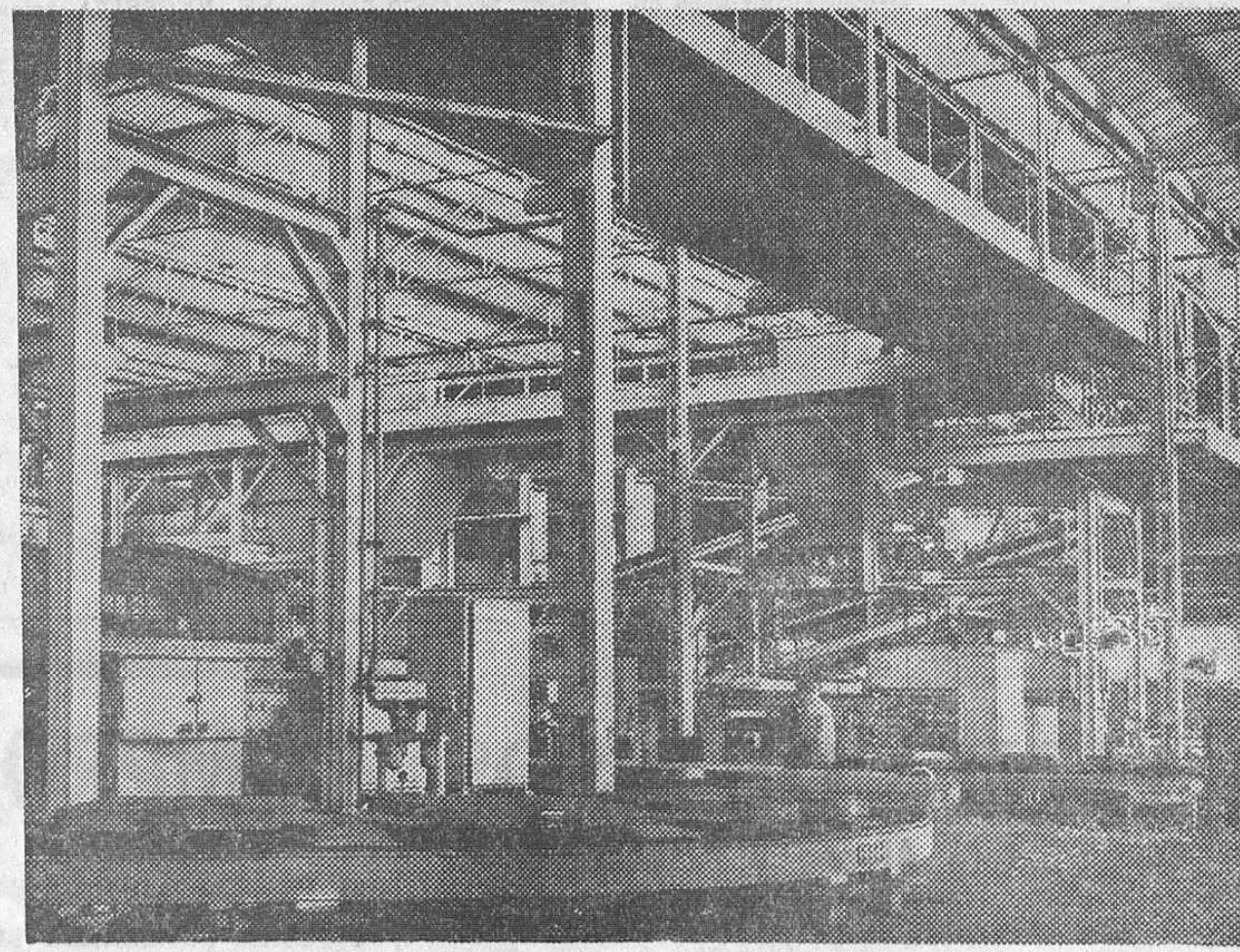
VISTA PARCIAL DE LAS INSTALACIONES DE LA NUEVA PLANTA AUTOMATICA PARA LA FABRICACION DE RADIADORES DE FUNDICION INAUGURADA RECIENTEMENTE
