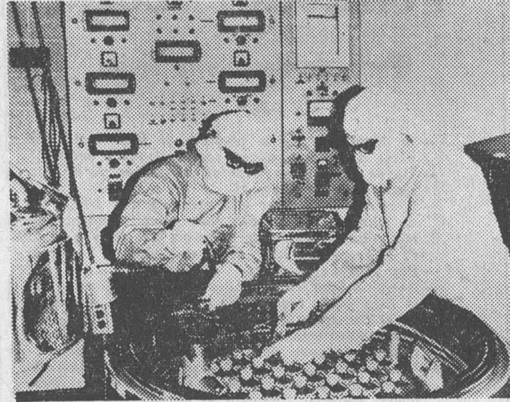
Secador en vacío para la obtención de plasma sanguíneo. (Foto Fiel)
