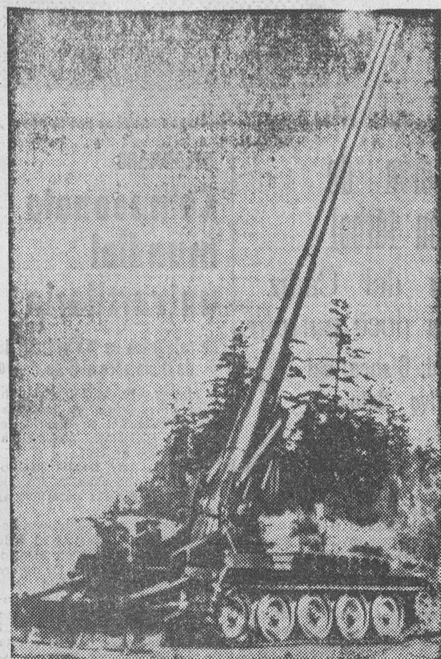
El gigante de la artillería del Ejército de los Estados Unidos, el cañón autopropulsado de 175 milímetros "M-107", durante una demostración del Departamento de Defensa norteamericano.
