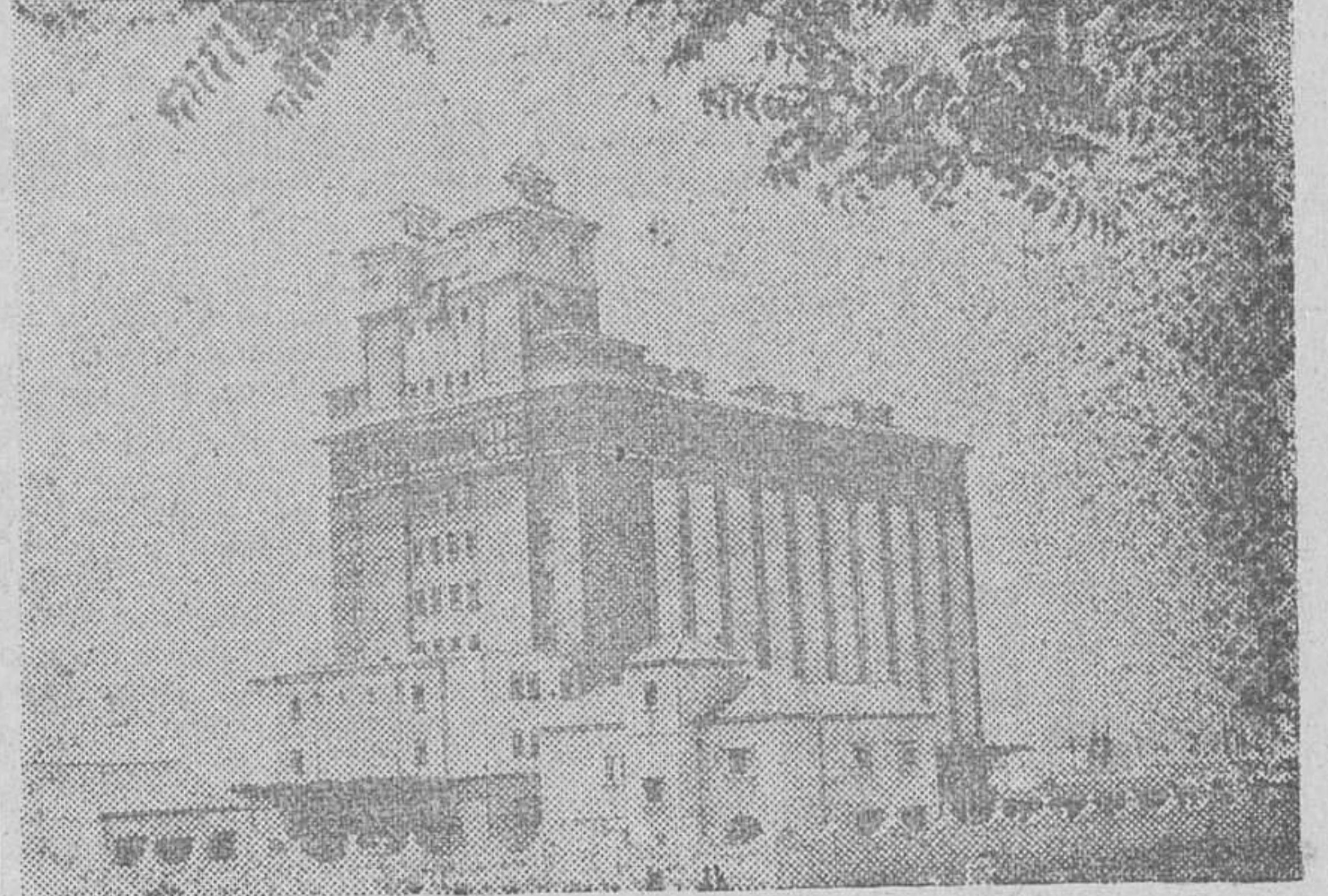
VISTA DEL SILO PARA CEREALES INAUGURADO POR S. E. EL JEFE DEL ESTADO EN CORDOBA. ES EL SILO MAS IMPORTANTE DE TODA LA RED NACIONAL QUE SE ESTA CONSTRUYENDO. — Foto CIFRA GRAFICA
