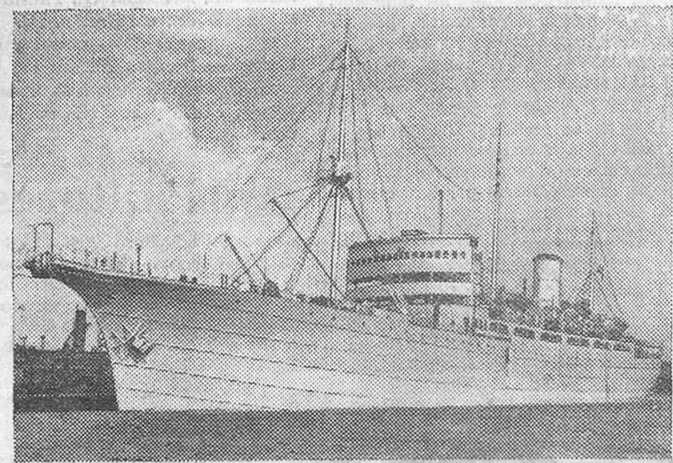
Vista del "Monarch", buque cablero recientemente puesto en servicio por la Dirección General de Comunicaciones de Inglaterra. Es el mayor de su clase en el mundo y va provisto de aparatos y dispositivos modernos para el tendido y reparación en alta mar de los cables submarinos (Foto Calpe)
