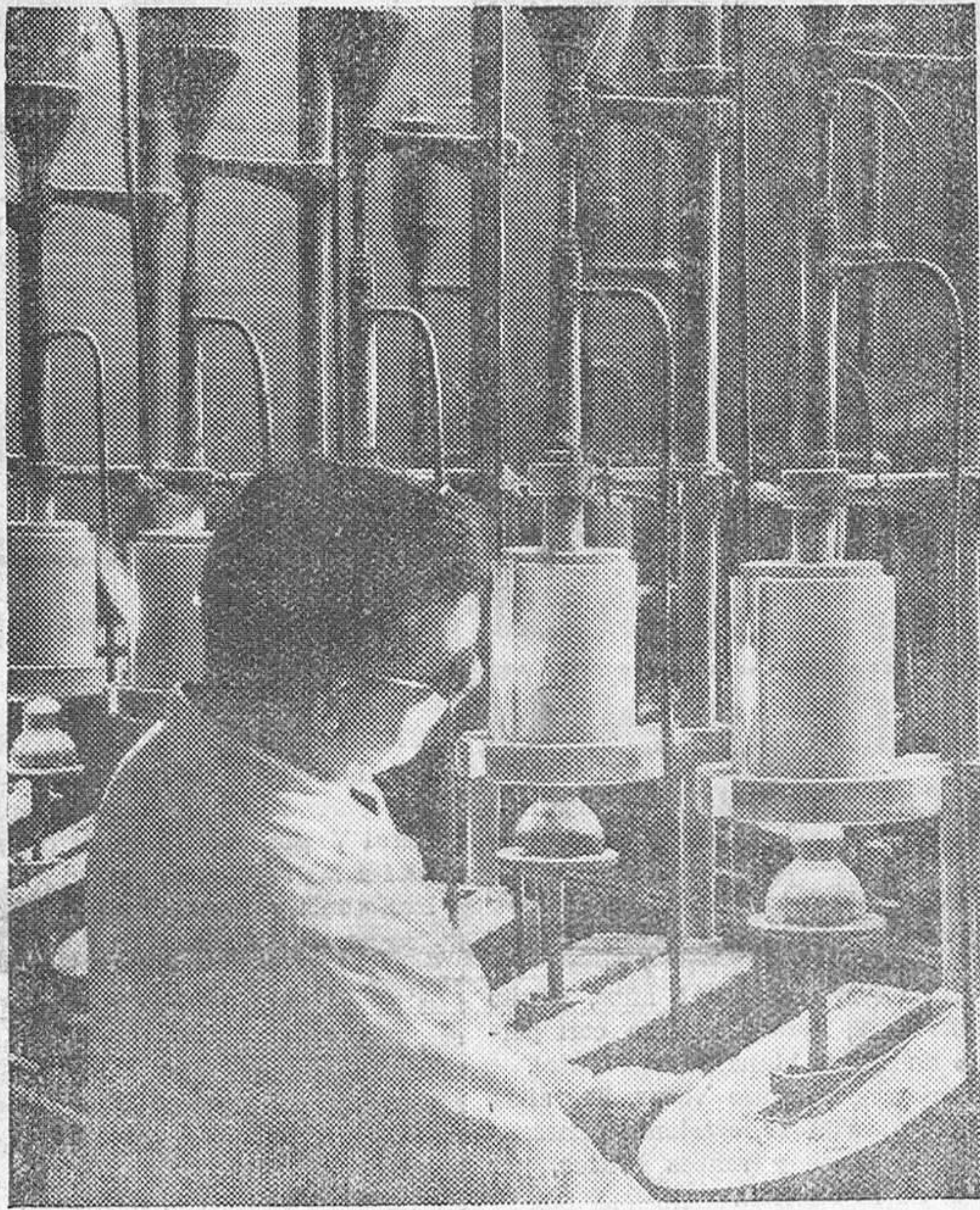
La "mepacrina" es un producto químico sustitutivo de la quinina, que ha sido empleado con notable éxito para combatir el paludismo. La máquina que aparece en la fotografía, puede fabricar 340 tabletas de este producto por minuto y en la fábrica inglesa donde está instalada aquélla se producen semanalmente 40 millones de pastillas. (Foto Calpe)
