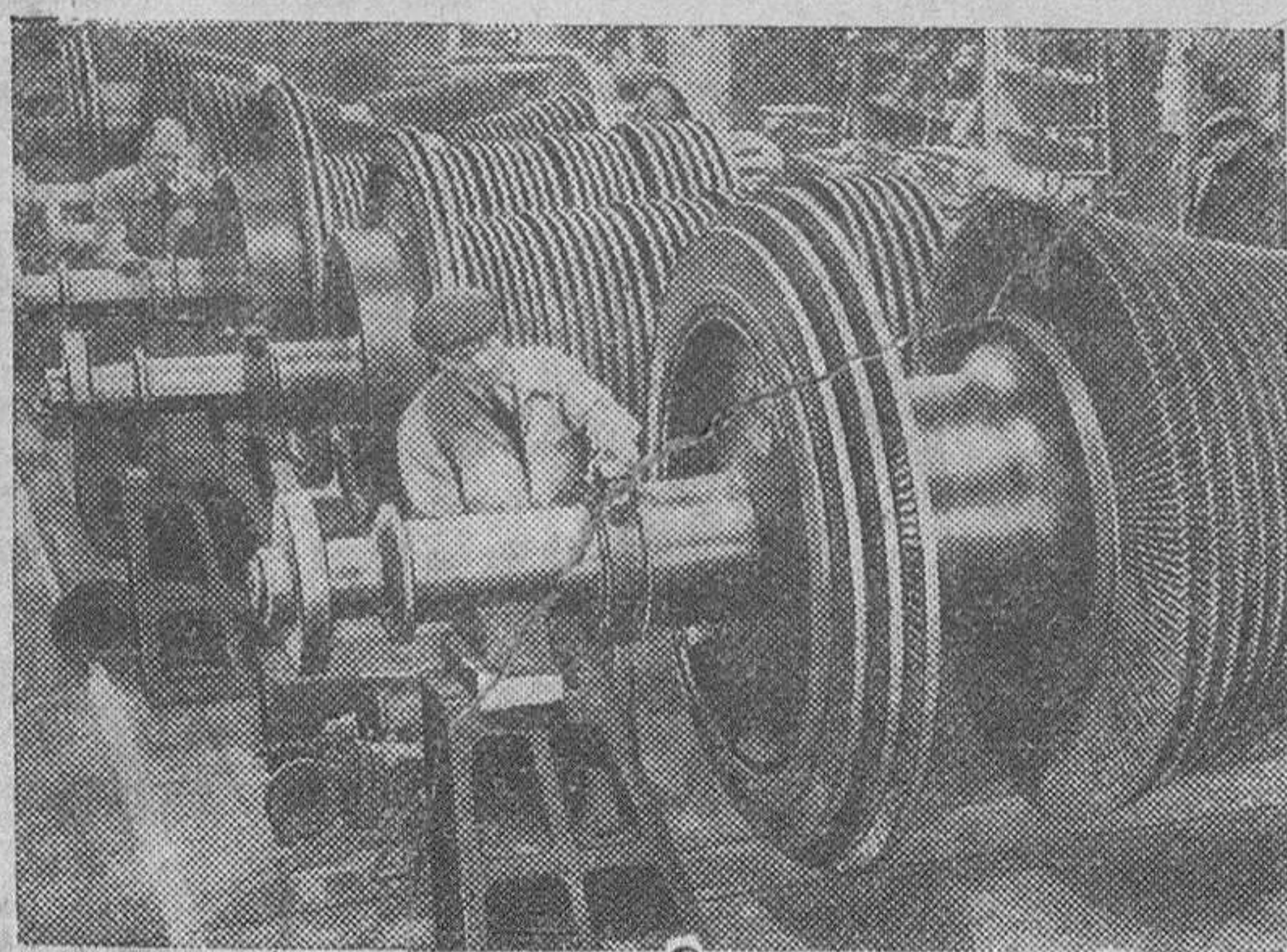
Un aspecto de la nave de turbinas en los talleres de Vickers-Armstrong, en Barrow-in-Furness, Inglaterra
