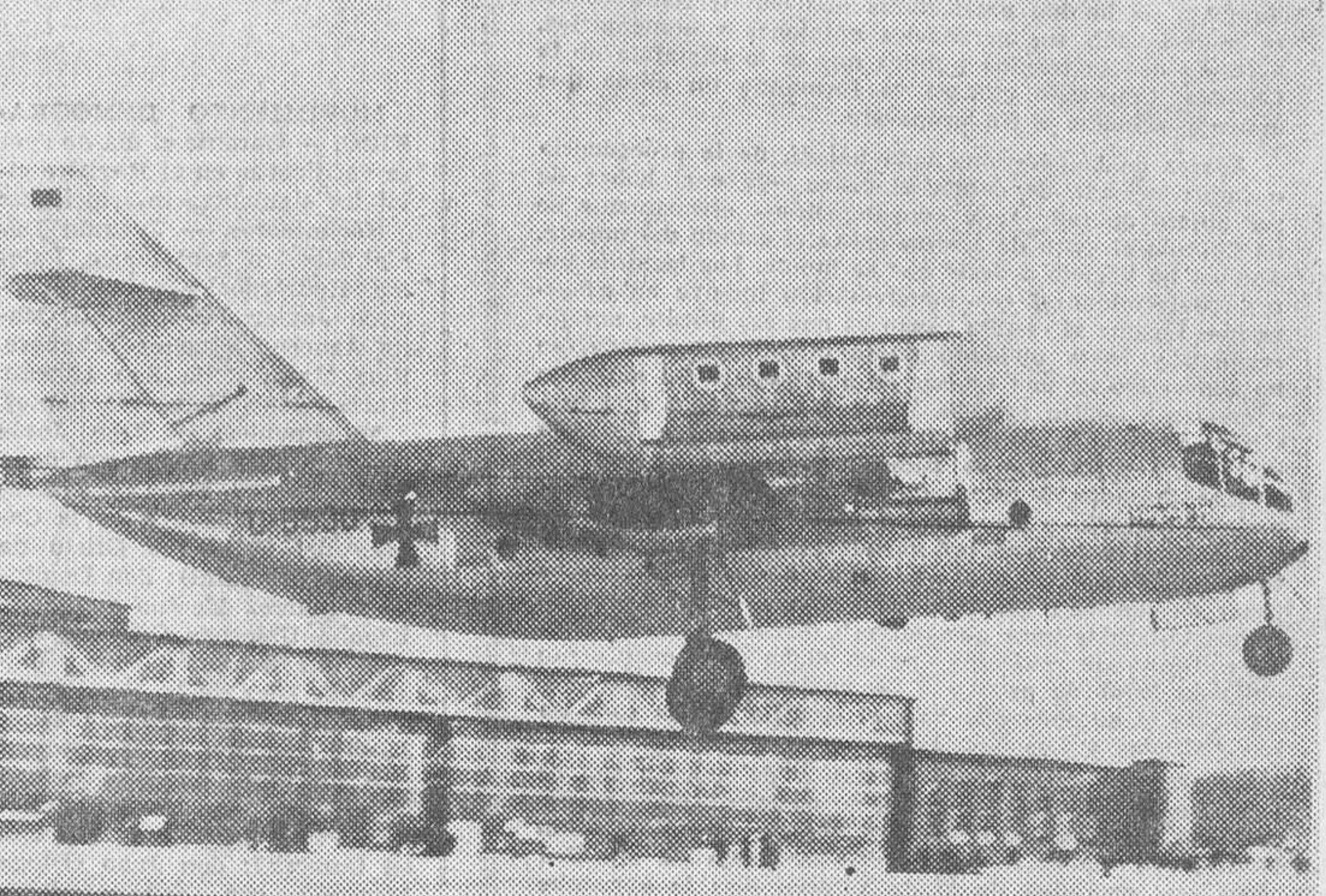
Munich (Alemania). — La NASA parece interesada en el avión de despegue vertical «DO-31» de la Dornier Company de Alemania occidental. En la fotografía, uno de estos aparatos durante una demostración en el aeropuerto de Oberpfaffenhofen, cerca de Munich. — (Telefoto UPI-CIFRA).
