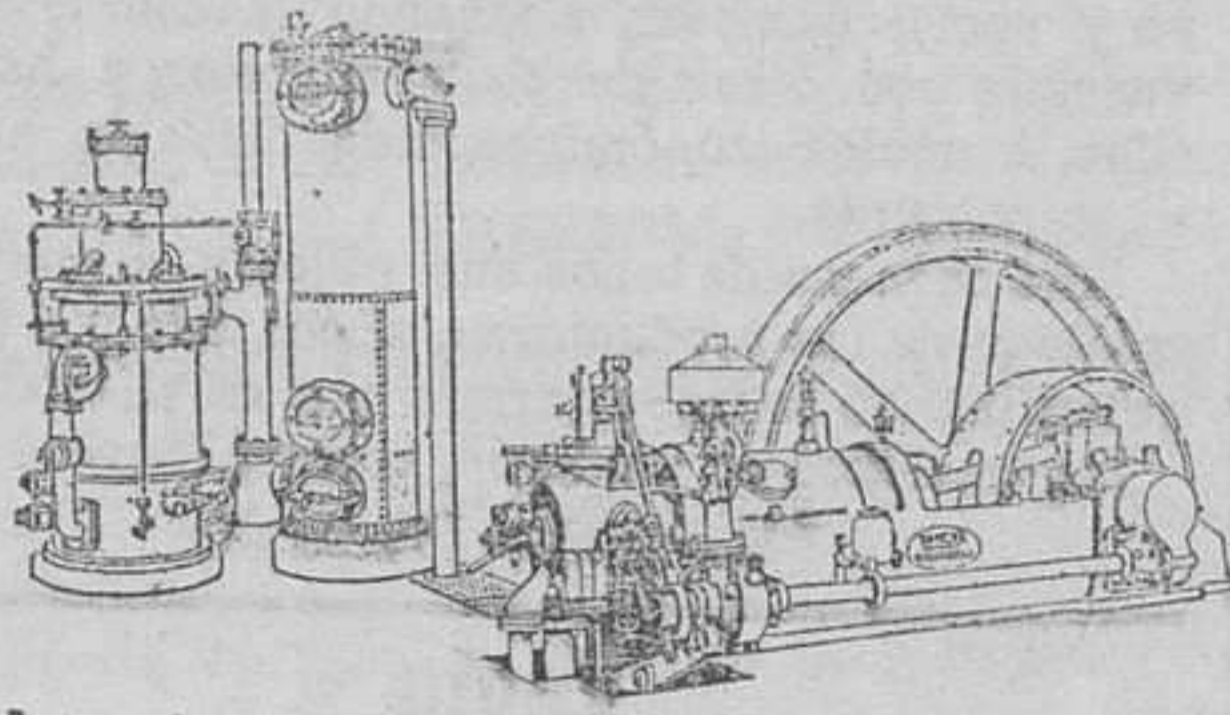
Motor de Gas Pobre por Aspiración «Tangyess»
