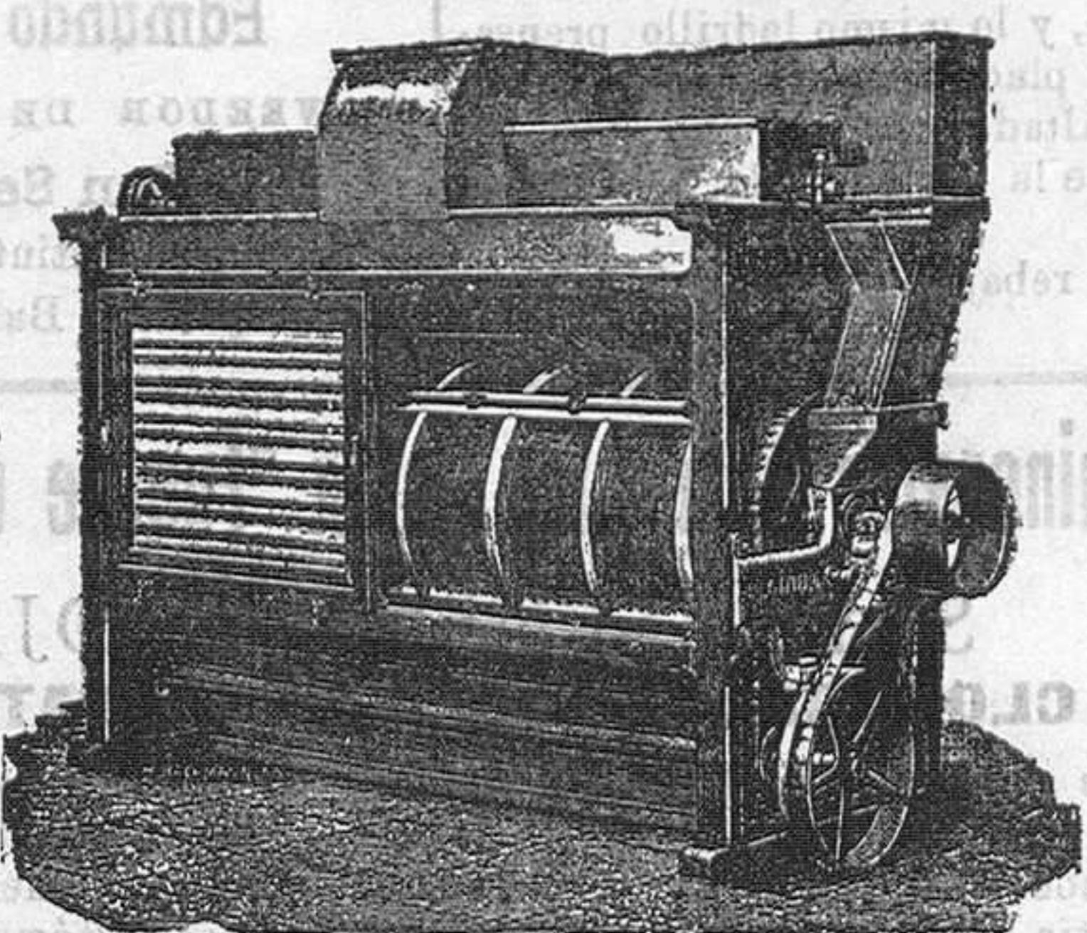
COLUMNA DESPUNTADORA
