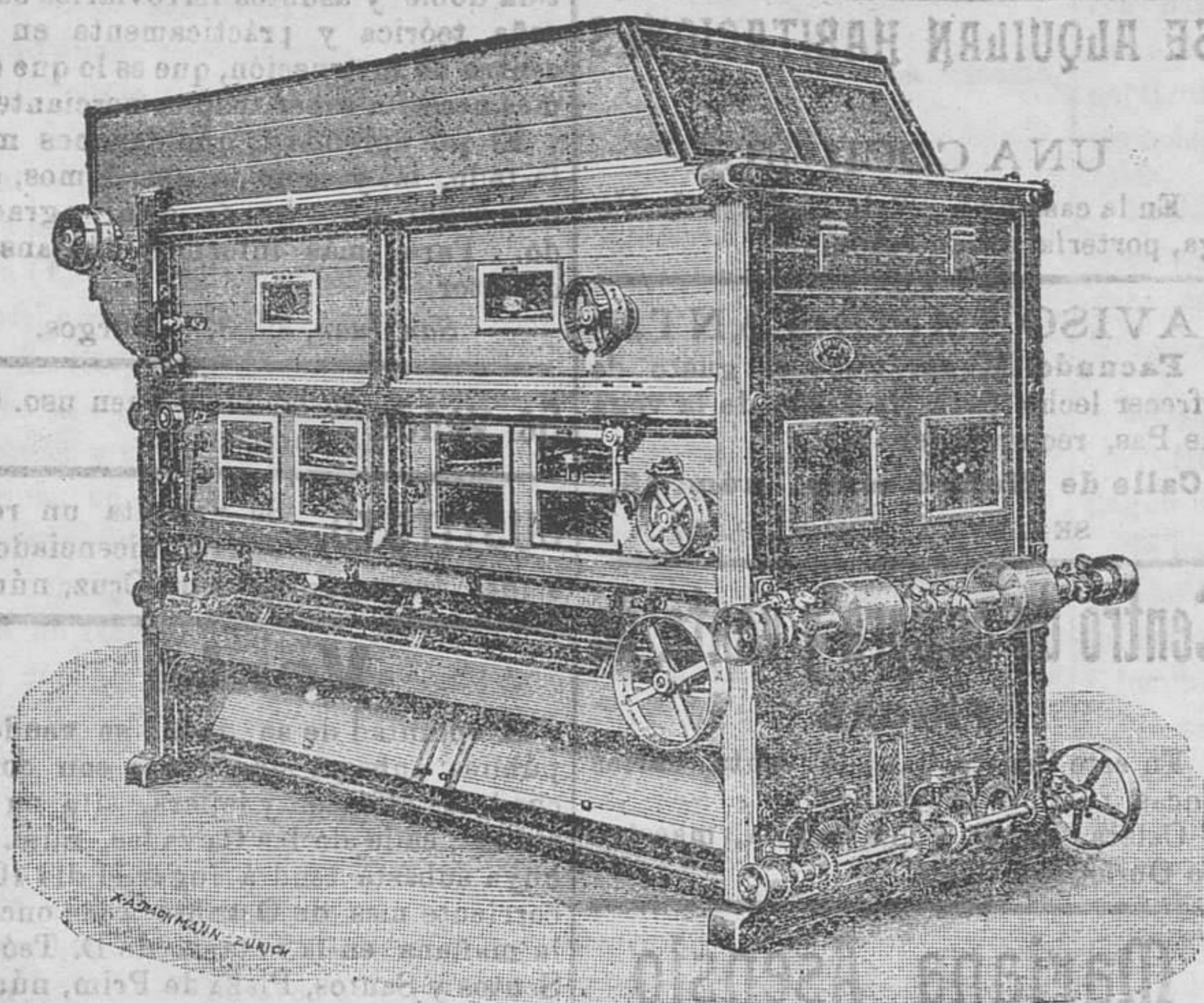
COLUMNA DESPUNTADORA
